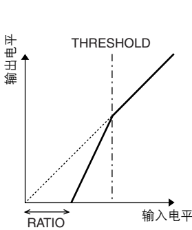
I/O 特征 (KNEE= 硬, OUT GAIN=0.0dB)
