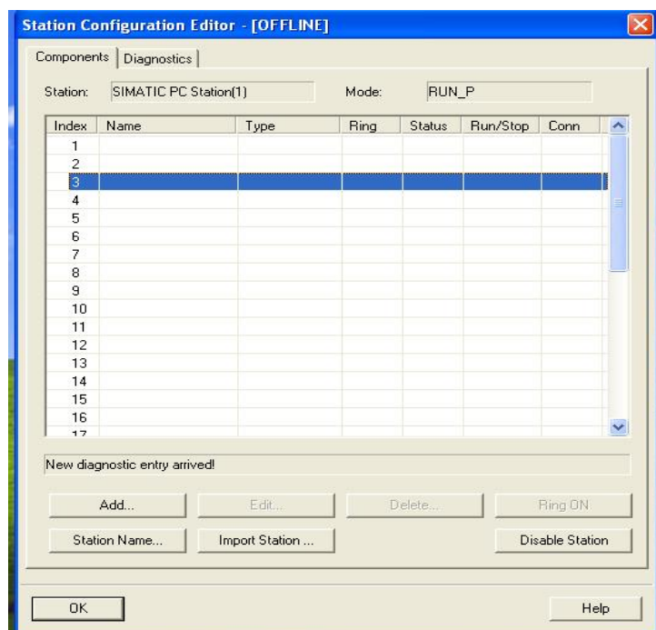
图 3: Station Configuration Editor 配置窗口
