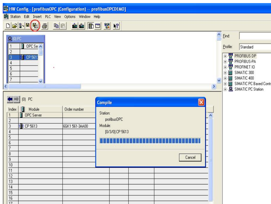
图 13: 组态的编译存盘
