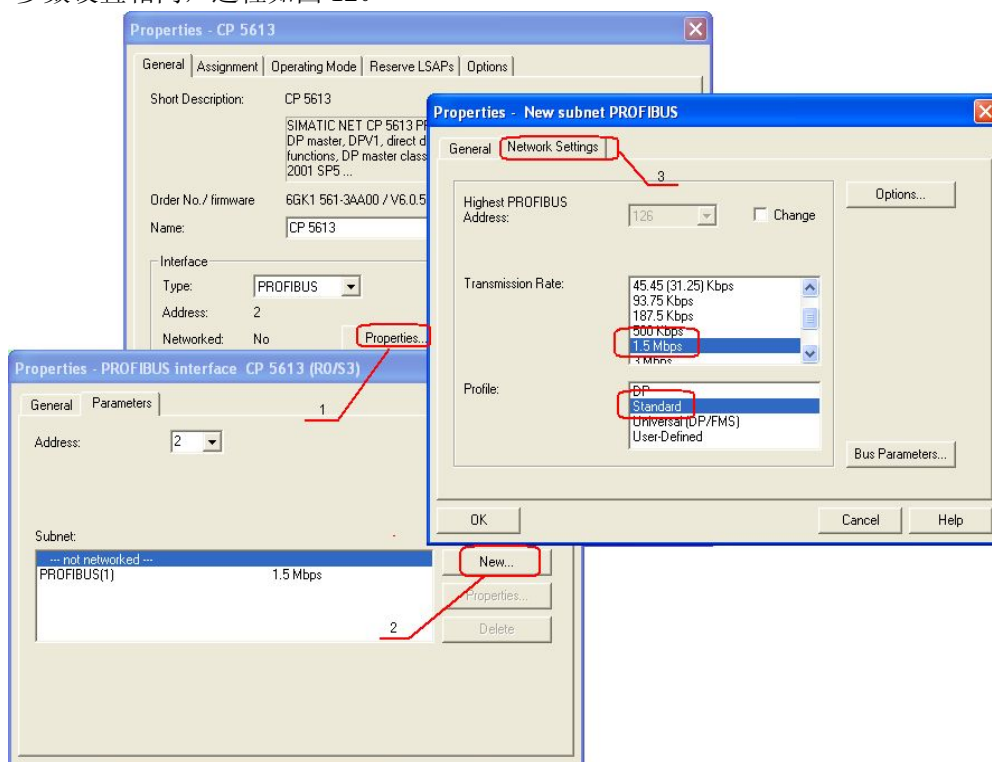
图 12: CP5613 参数设置
