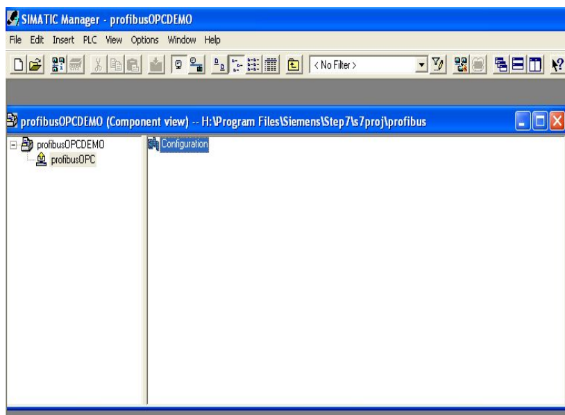
图 10： STEP 7 中创建新项目与建立 Simatic PC Station
