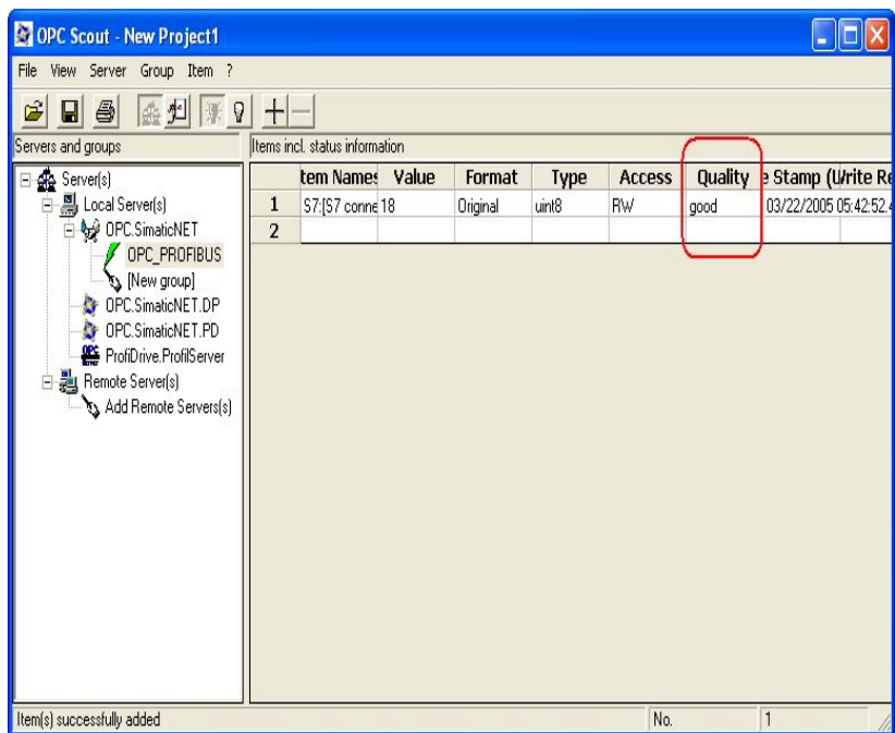
图 25： OPC Scout 与 OPC Server 的连接
