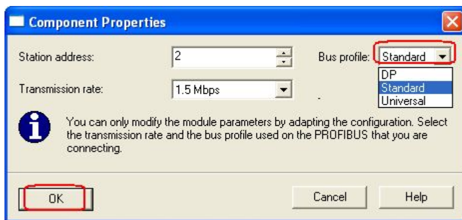
图 6： 分配 CP5613 参数
