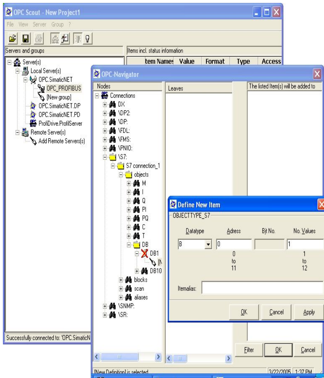
图 23: 定义条目及标签变量
