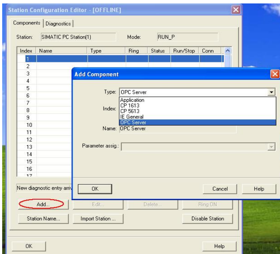
图 4: 添加 OPC Server
