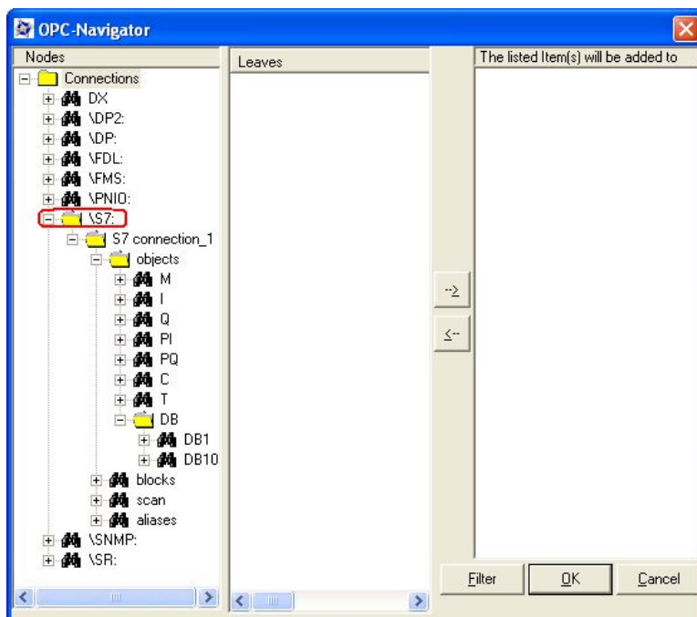
图 22: OPC Navigator 中的对象
