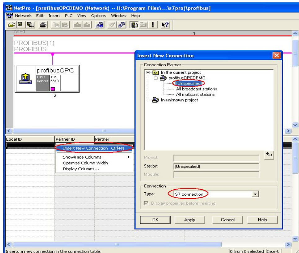
图 16：在网络配置（NetPro）中添加新连接
