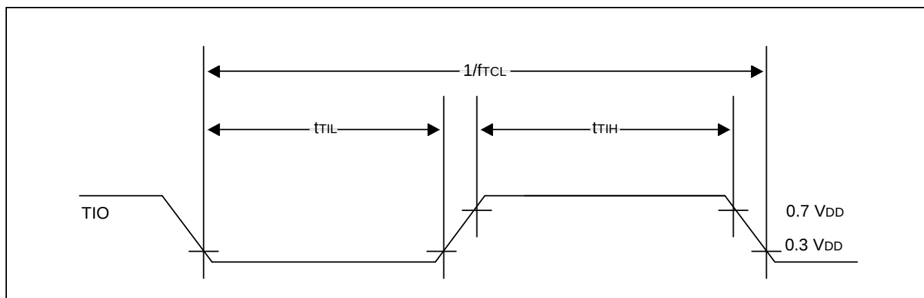
Figure 14-6. TIO Timing
