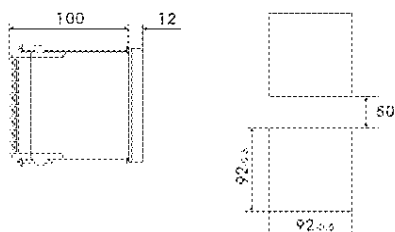
开孔尺寸
