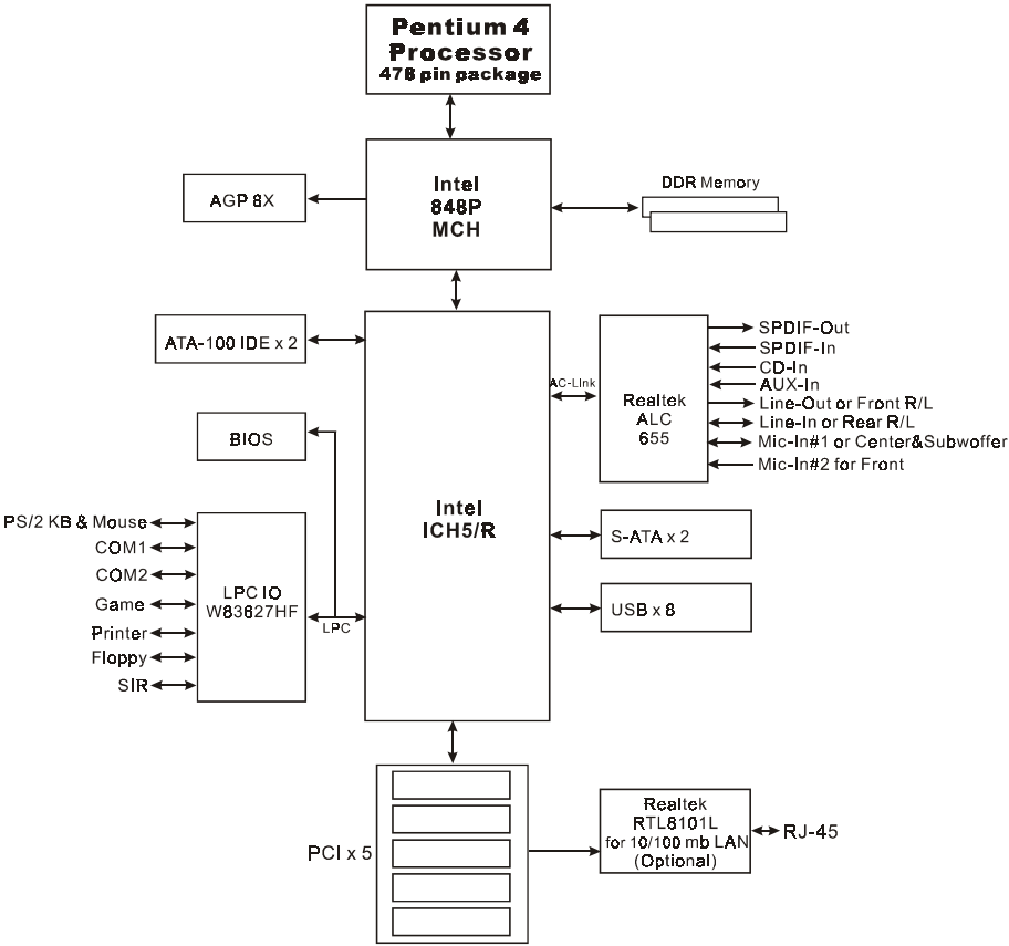
<图5> 系统方块图
