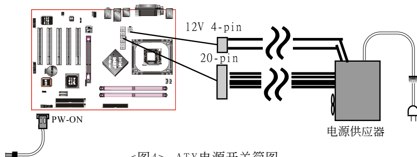
<图4> ATX电源开关简图
