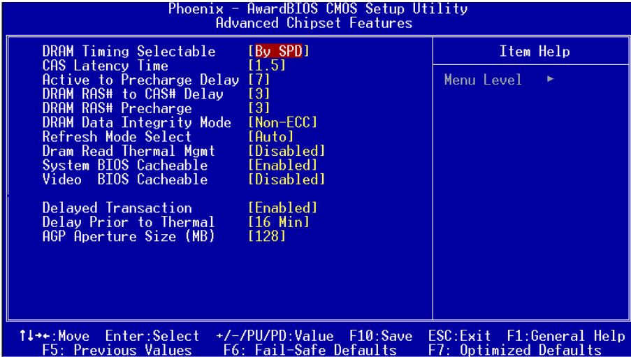
图4-4 芯片组高级设置
