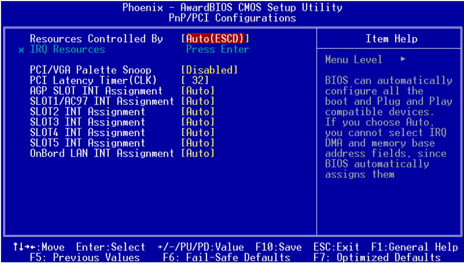
图4-7 即插即用/PCI装置设定
