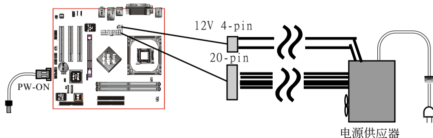
<图4> ATX电源开关简图
