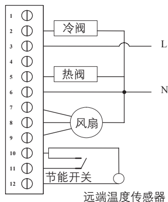
VC4013阀接线图
