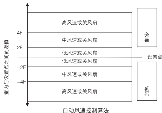
自动风速控制算法
