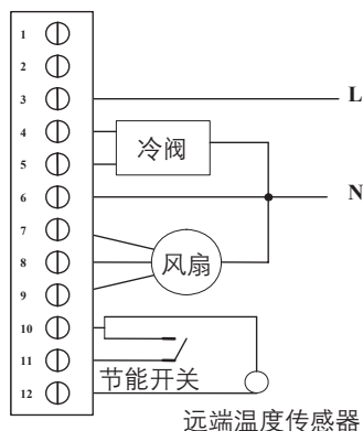
VC6013阀接线图
