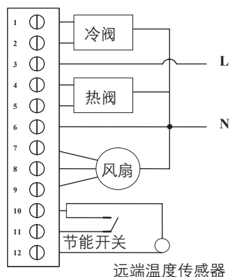
VC6013阀接线图
