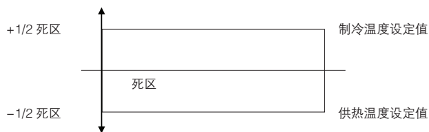
四管制自动冷热切换算法
