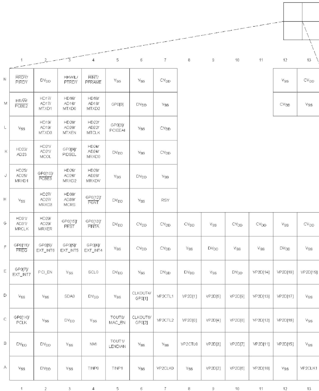
图 2-5 DM642 引脚映射 (C 象限)
