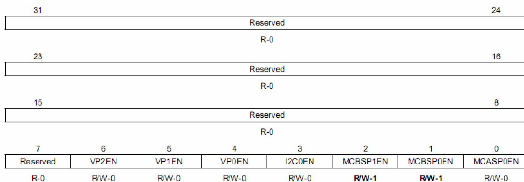
图 3-1, 外设配置寄存器 (PERCFG)
