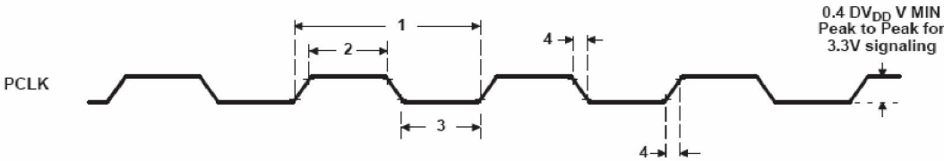
图 5-46 PCLK 时序
