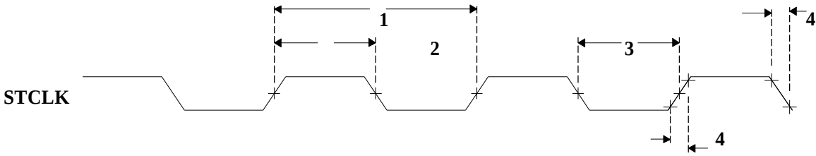
图 5-62.STCLK 时间
