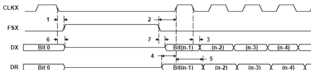
图 5-54 MCBSP 时序 当 SPI 为主或从模式时 \text{CLKSTP} = 11b, \text{CLKXP} = 0
