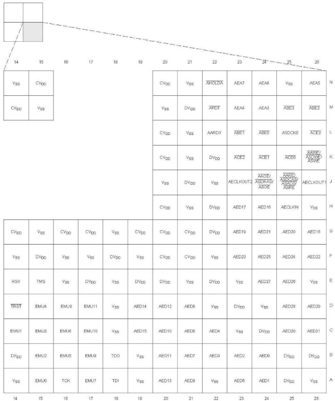
图 2-6 DM642 引脚映射 (D 象限)
