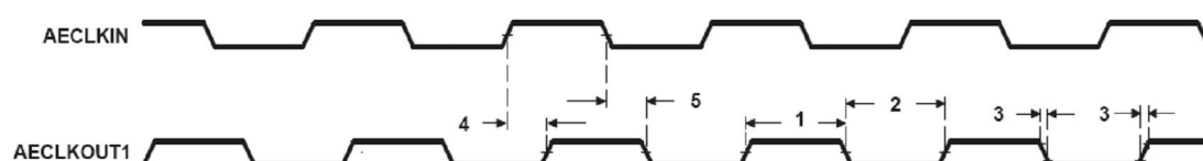
图 5- 15 BMIFA 模块的 AECLKOUT1 时序
