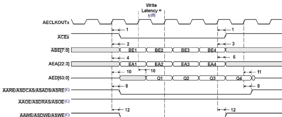
图 5-20 EMIF模块的可编程同步接口写时序 (写等待=0) (A) (B)
