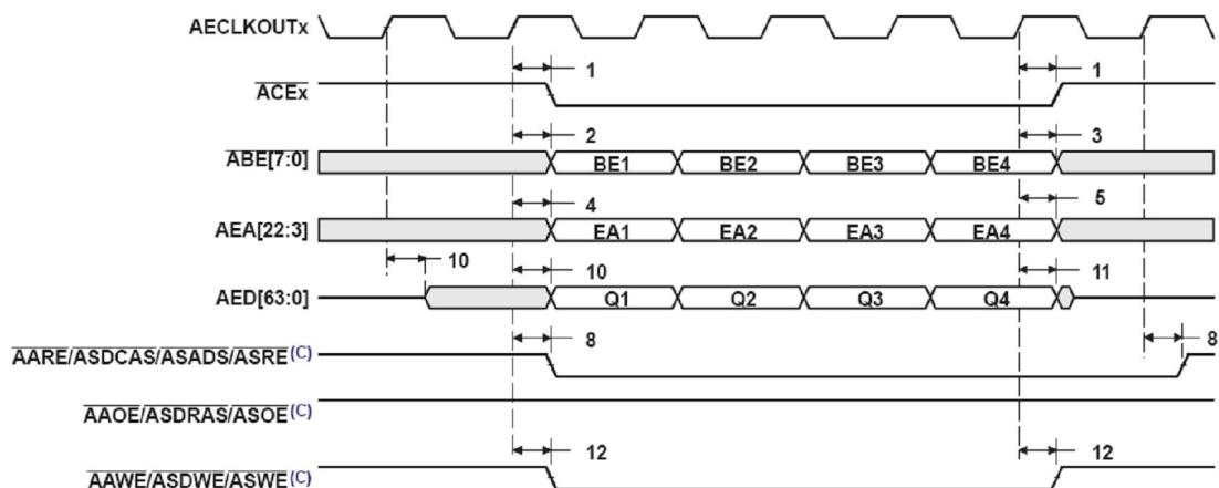
图 5-19 BIFACE 模块的可编程同步接口读时序 (读等待 = 2) (A) (B)
