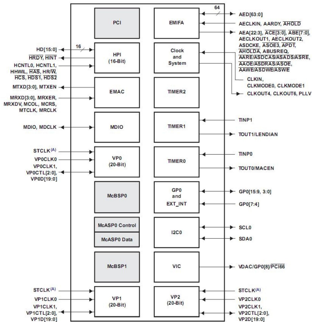
图 3-6 到图 3-8 列举了 DM642 可配置外设的例子。
