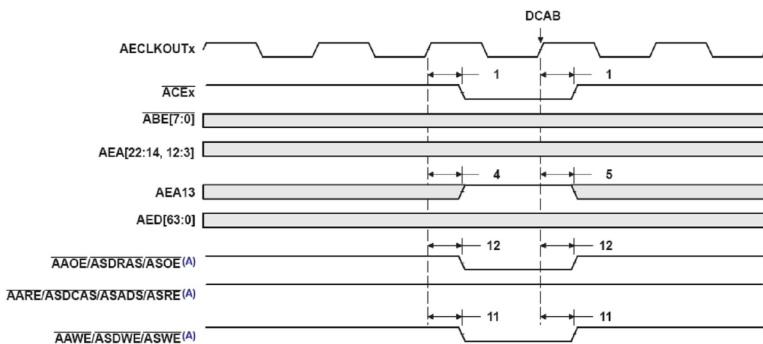
图 5- 24 EMIFA 模块 SDRAM ACTV 控制时序
