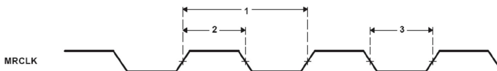
图 5-63. MRCLK 时序 (EMAC - 接收)
