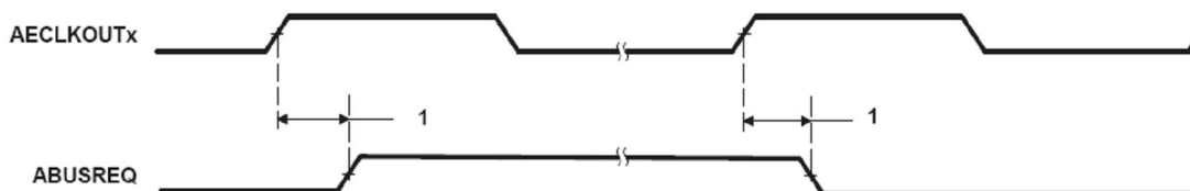
图 5-31 EMIFA 模块的 BUSREQ 时序
