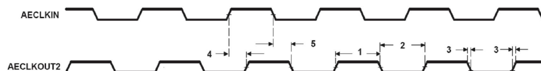
图 5- 16 BMIFA 模块的 AECLKOUT2 时序
