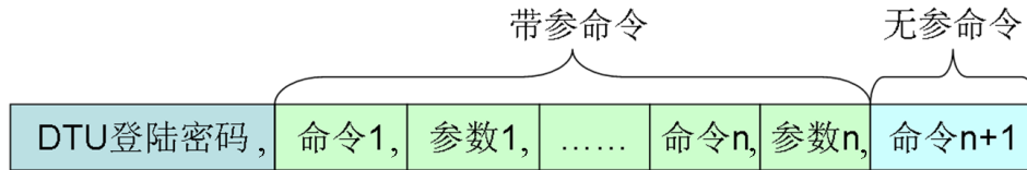
图 3.9 短信配置命令格式
