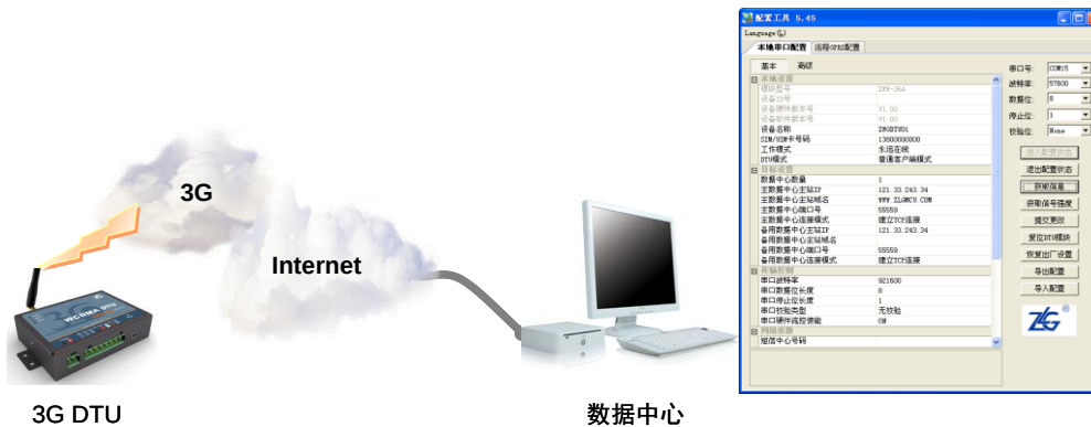
图 3.5 远程配置示意图
