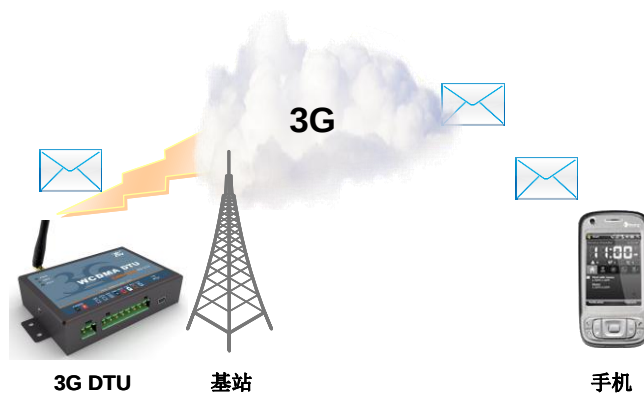
图 3.8 短信配置示意图
