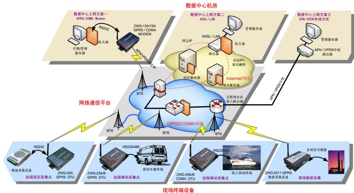
图 2.1 组网方案示意图
