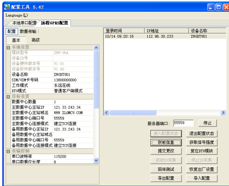
图 3.7 远程配置获取信息界面
