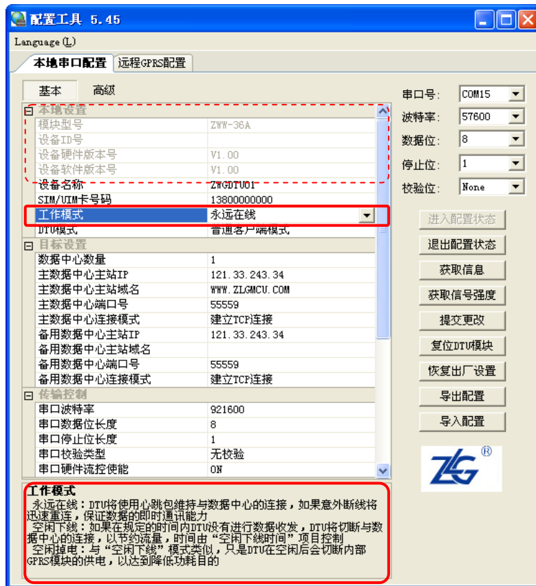
图 3.4 配置界面
