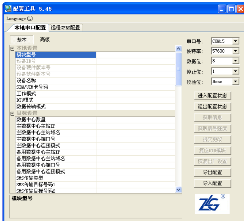
图 3.3 ZWW-36A 配置界面
