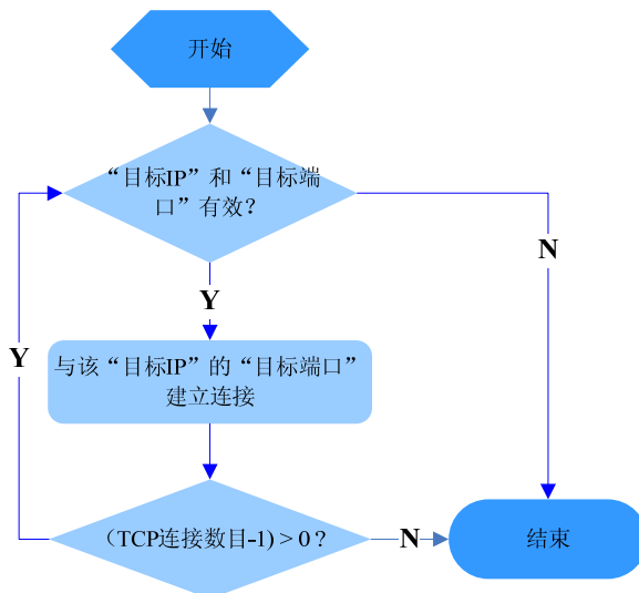
图 6.14 ZNE-100TL 模块在 TCP Client 模式下建立连接流程
