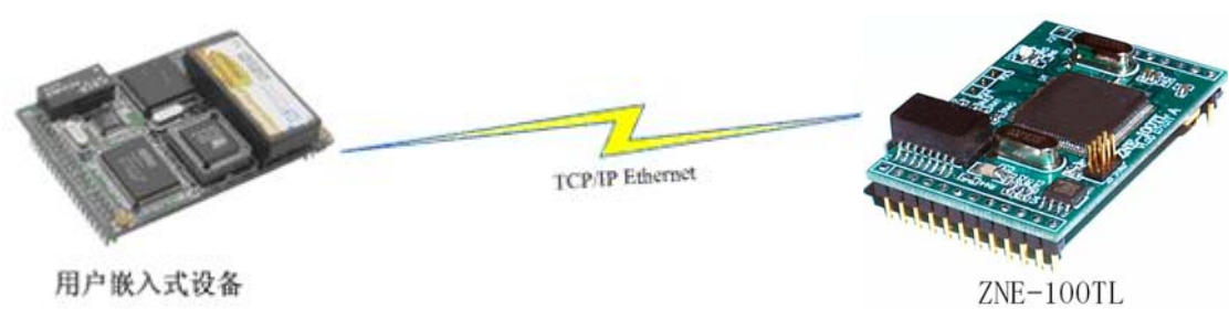
图 6.15 用户设备使用 TCP 连接方式配置 ZNE-100TL 模块
