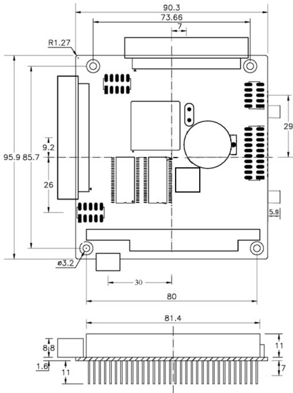
图 5.2 EPC-8000A 工控机主板机械尺寸
