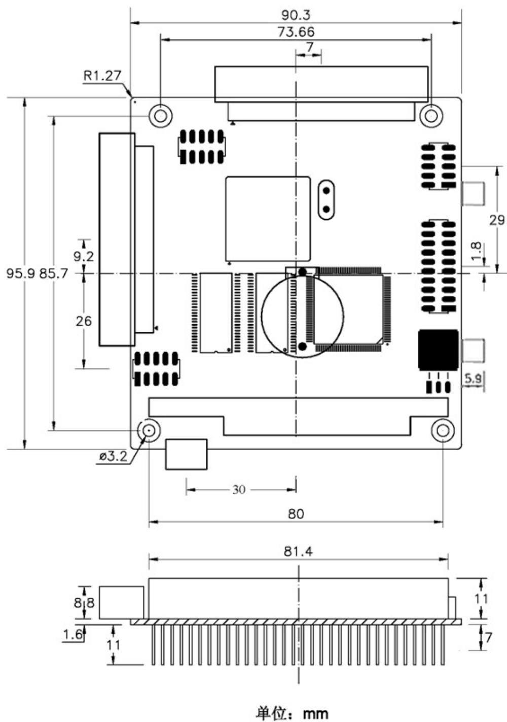
图 5.1 EPC-8000 工控机主板机械尺寸
