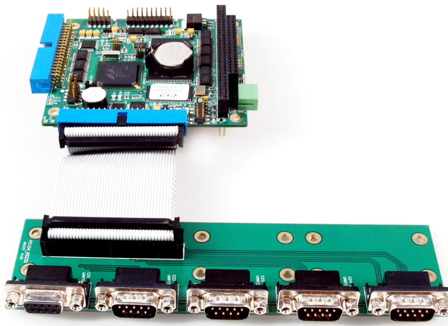
图 4.1 PC104_RS232 板与 EPC-8000 连接图
