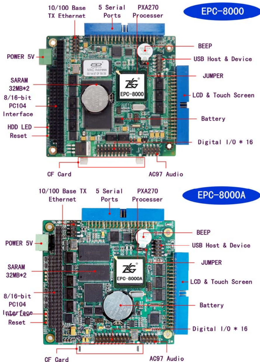
图 1.1 EPC-8000 工控机主板
