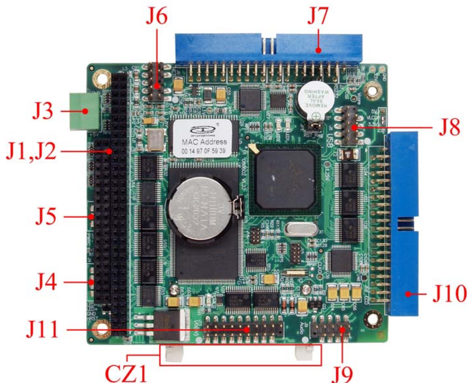
图 2.3 EPC-8000 工控机主板接口布局
