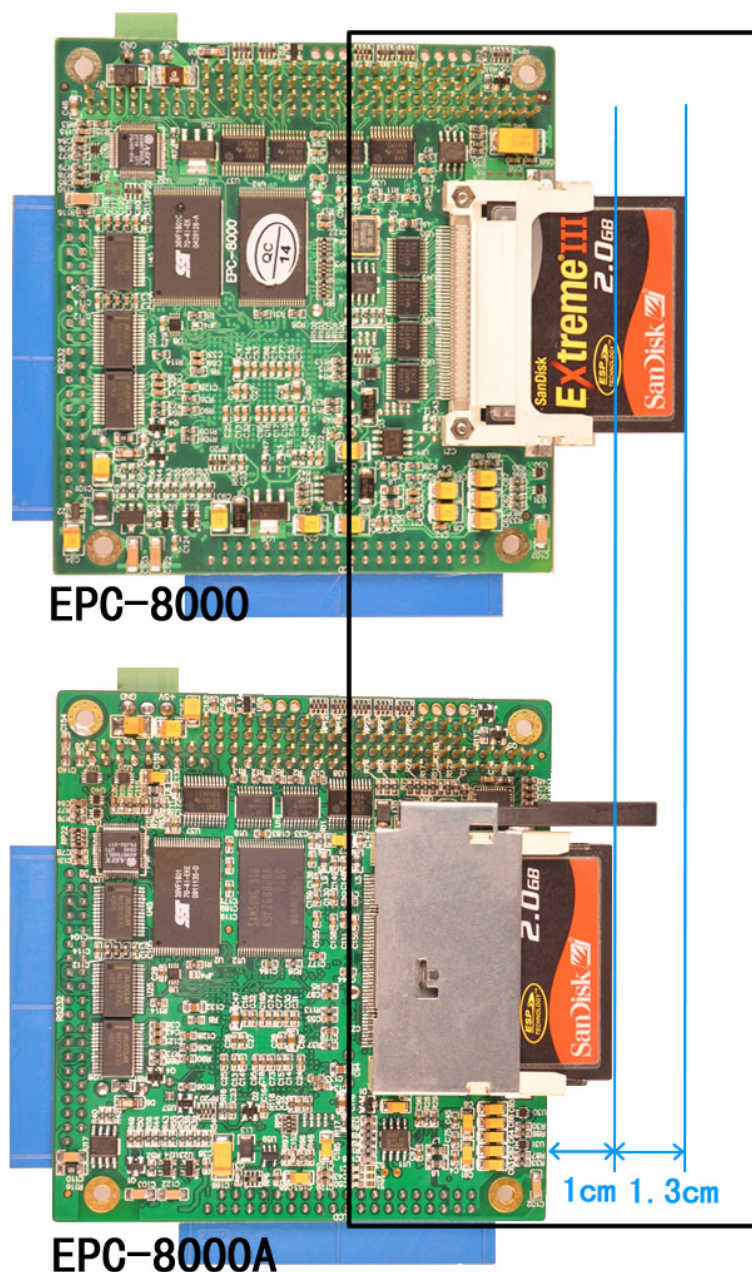
图 1.2 CF 卡的卡座的位置和外形
