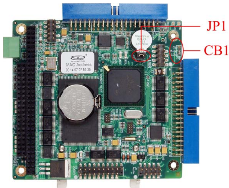
图 2.2 EPC-8000 工控机主板跳线器布局
