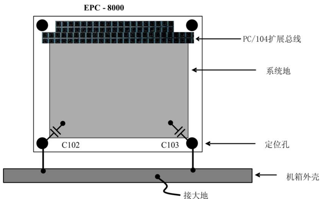
图 2.14 EPC-8000 工控机主板接地示意图
