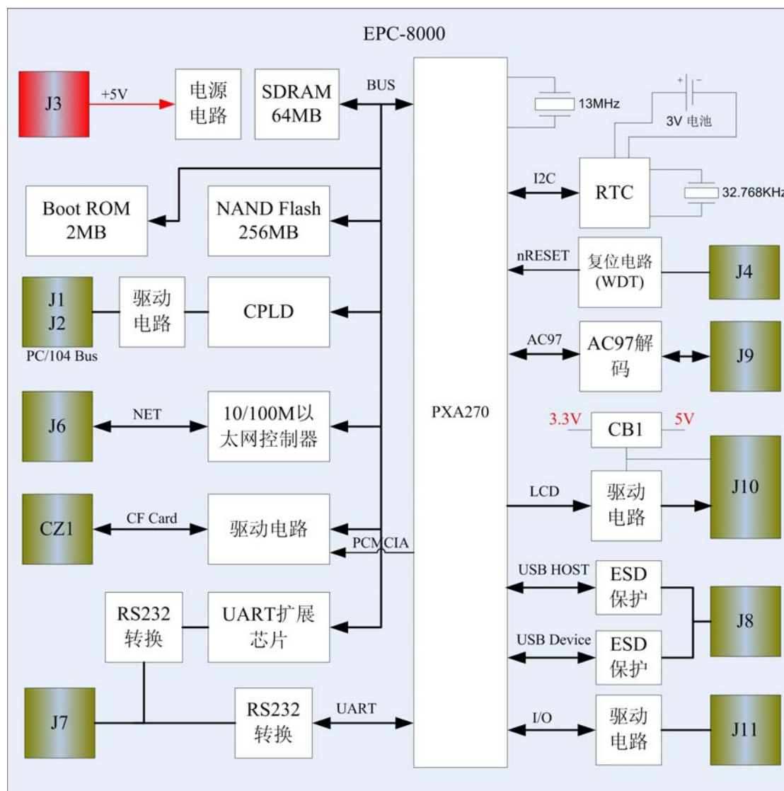
图 2.1 EPC-8000 工控机主板功能框图
