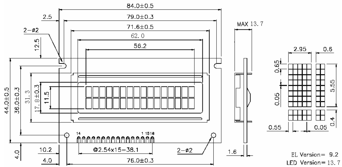
CM162-2 尺寸图：
