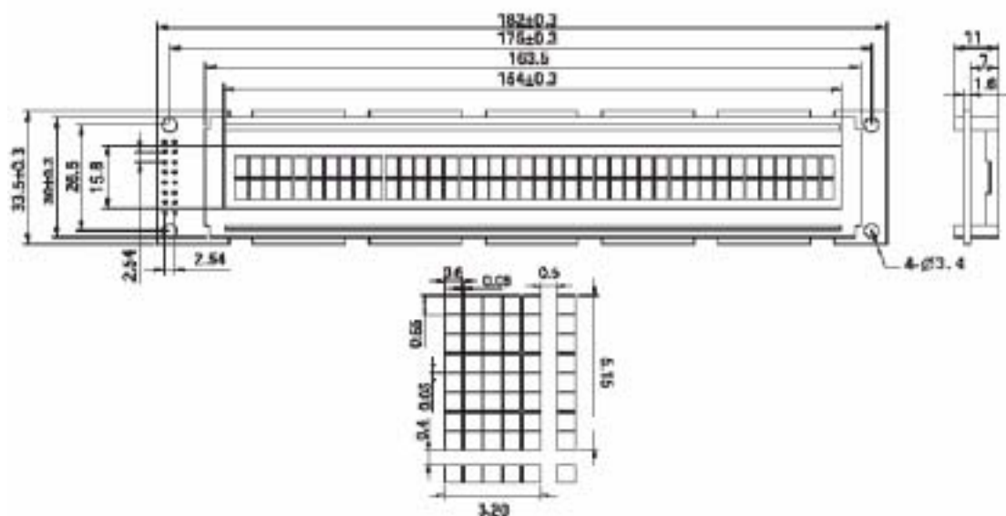
CM402-1 尺寸图：
