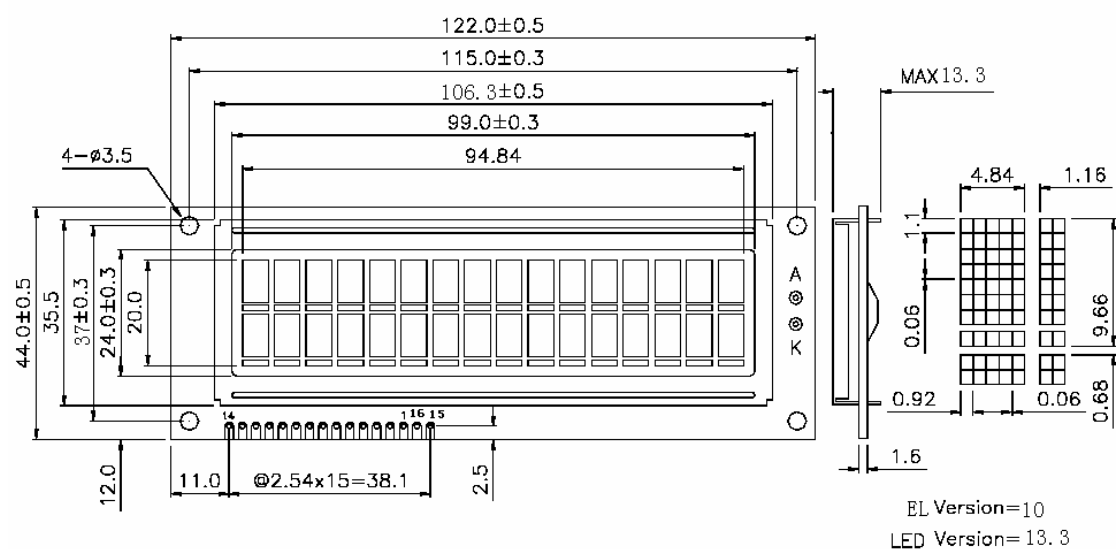
CM162-1 尺寸图：
