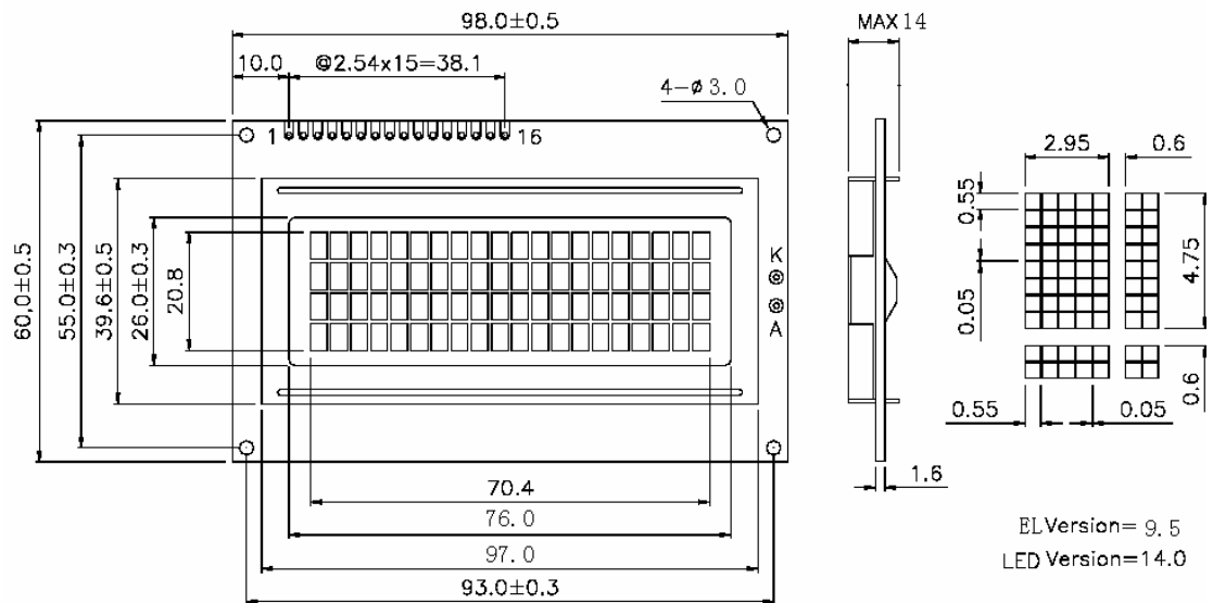
CM204-1 尺寸图：
