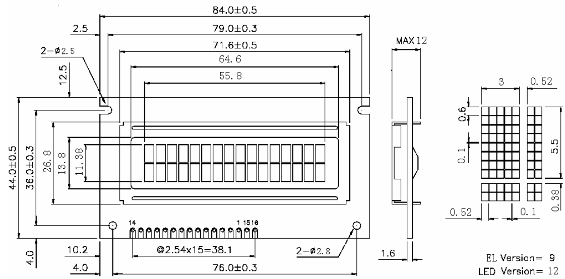
CM162-10 尺寸图：
