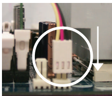
圖 2. 將 CPU 散熱風扇的電源線插入主機板上的 "CPU_FAN" 插座。
