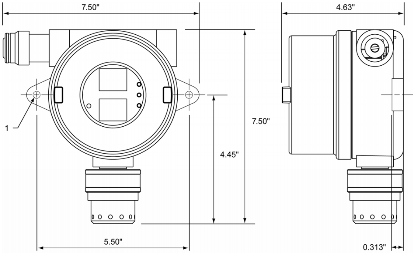
图4. 外形图
