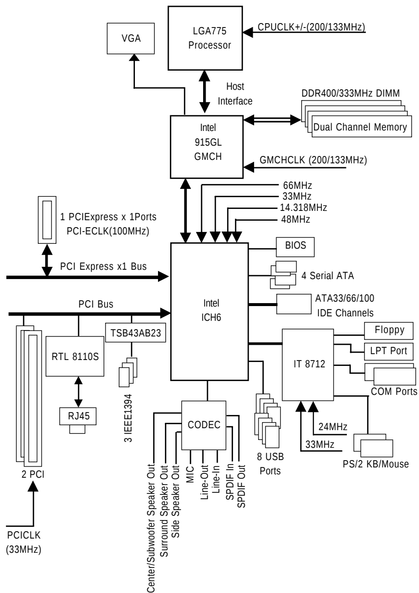
晶片組功能方塊圖
