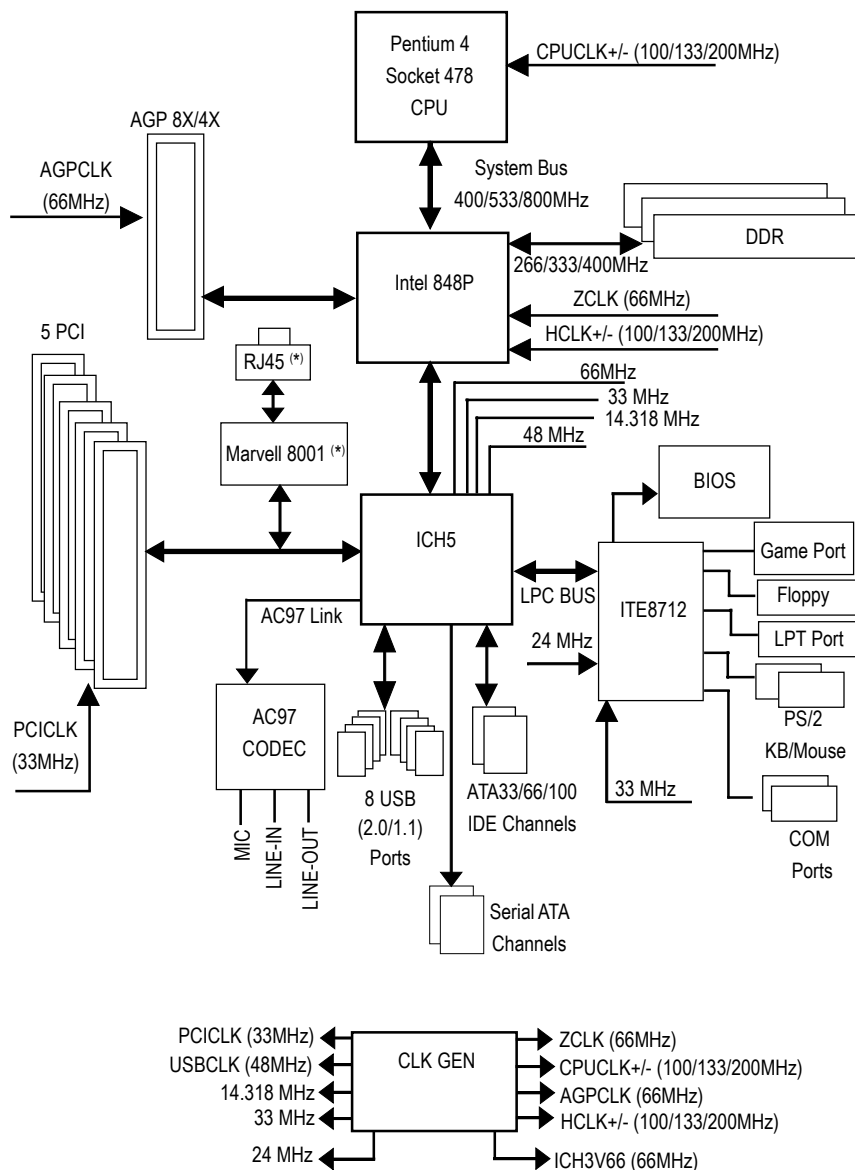
晶片組功能方塊圖
