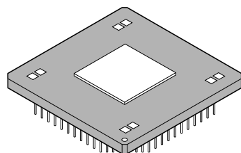
(PGA-401C-A02)
