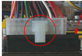
20-Pin 电源
