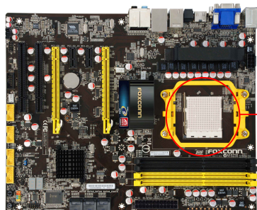
插座针脚1对应的边角
