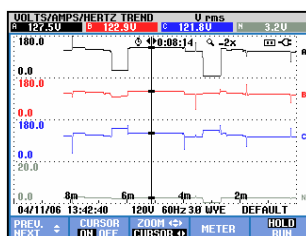
图 19-5. 趋势图显示（光标功能启用）
