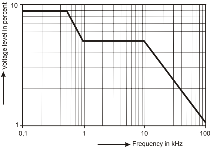
图 20-2. Meister Kurve（依照 EN50160）
