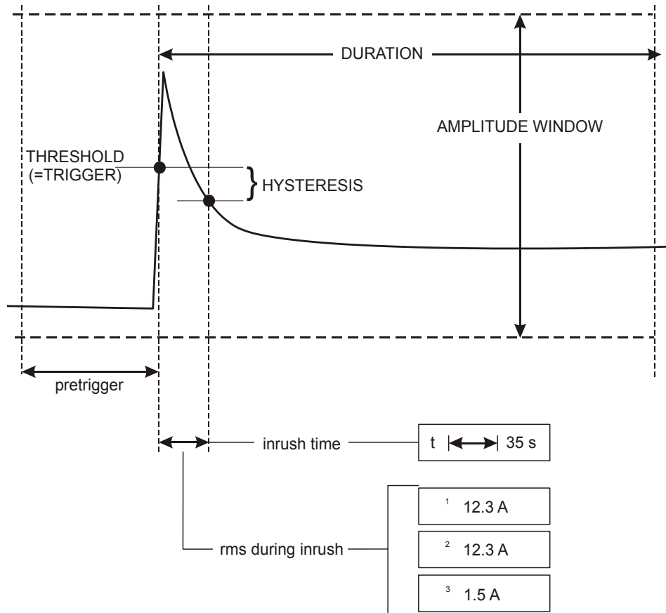
图 15-1. 浪涌特征及与开始菜单的关系
