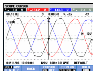
图 19-2. 波形显示（光标功能启用）
