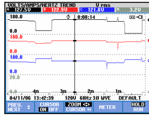
图 19-6. 趋势图显示（光标和缩放功能启用）
