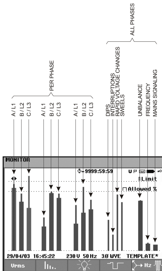
图 18-1. 电力质量监测主屏幕
