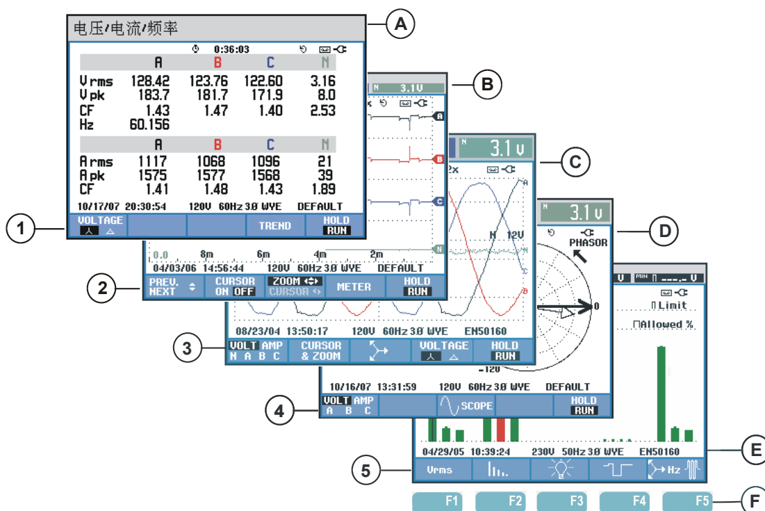
图 5-1. 显示类型概览
