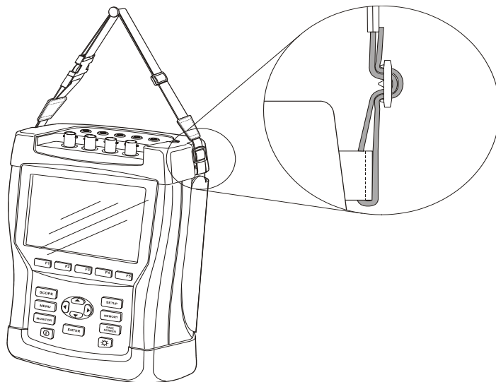
图 4-2. 固定挂带
