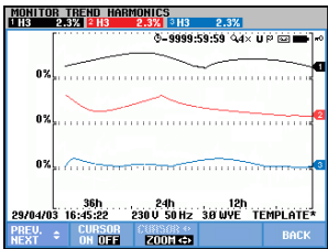
图 18-3. 趋势图显示
