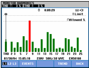
图 18-4. 条形图屏幕
