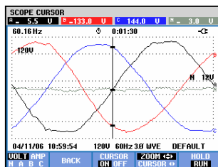
图 19-3. 波形显示（光标和缩放功能启用）
