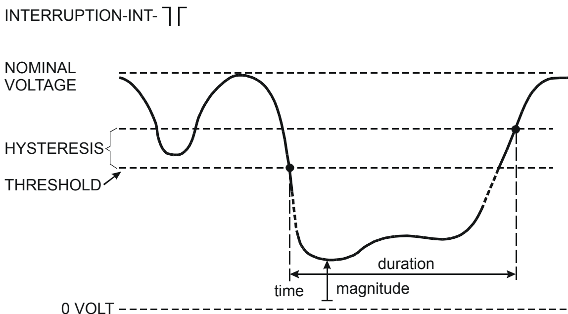
图 9-3. 电压干扰的特征
