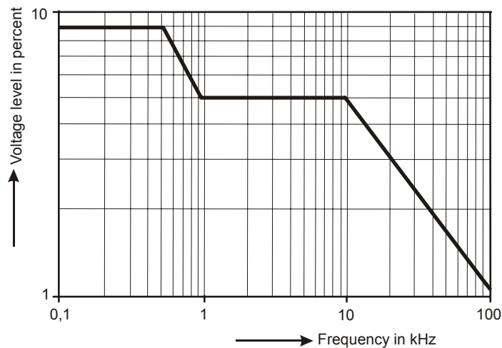
图 16-1. Meister Kurve（依照 EN50160）
