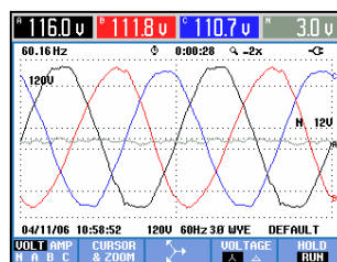
图 19-1. 波形显示（光标功能关闭）
