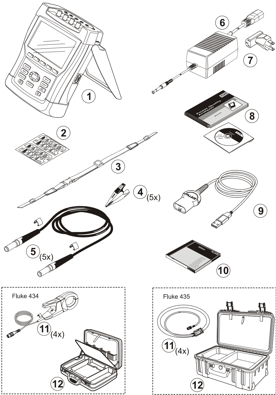
图 1-1. 分析仪套件的内容
