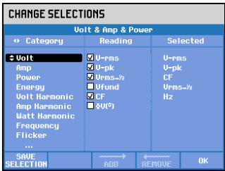
图 17-1.更改选择菜单
