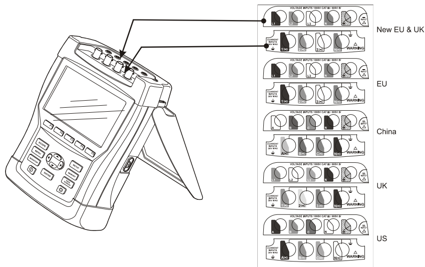
图 6-1. 安装电压和电流输入端贴纸
