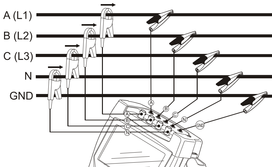
图 6-2. 将分析仪与三相配电系统连接
