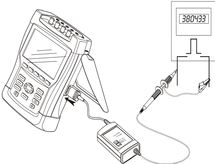
图 11-1. 利用脉冲输出验证能量计
