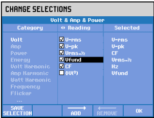
图 17-3.Vfund 可用于记录
