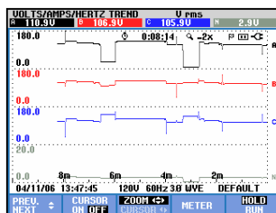
图 19-4. 趋势图显示（光标功能关闭）
