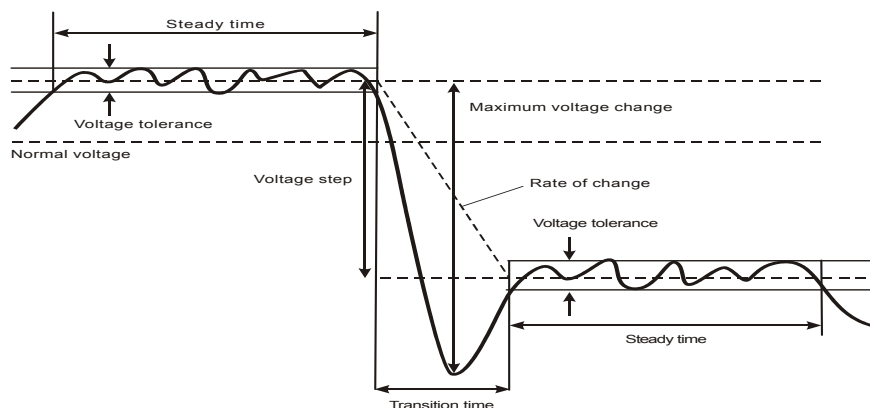
图 9-4. 快速电压变化的特征
