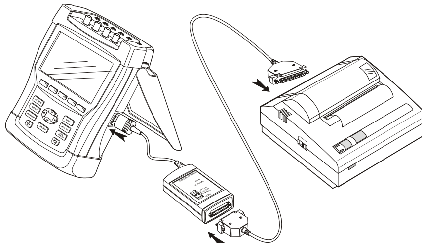
图 21-3. 分析仪，DPU-414 打印机和 PAC91 打印机转接器
