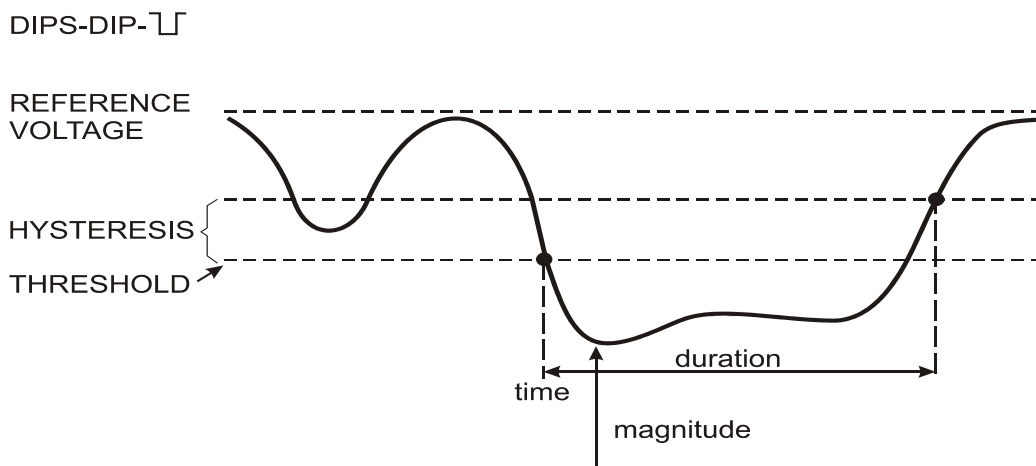
图 9-1. 电压骤降的特征
