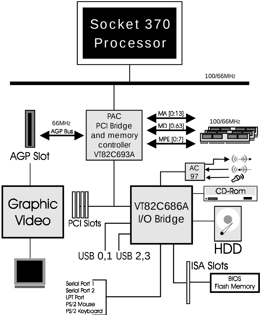
<圖5> 系統方塊圖
