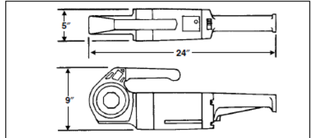
图 1-690 动力驱动尺寸
