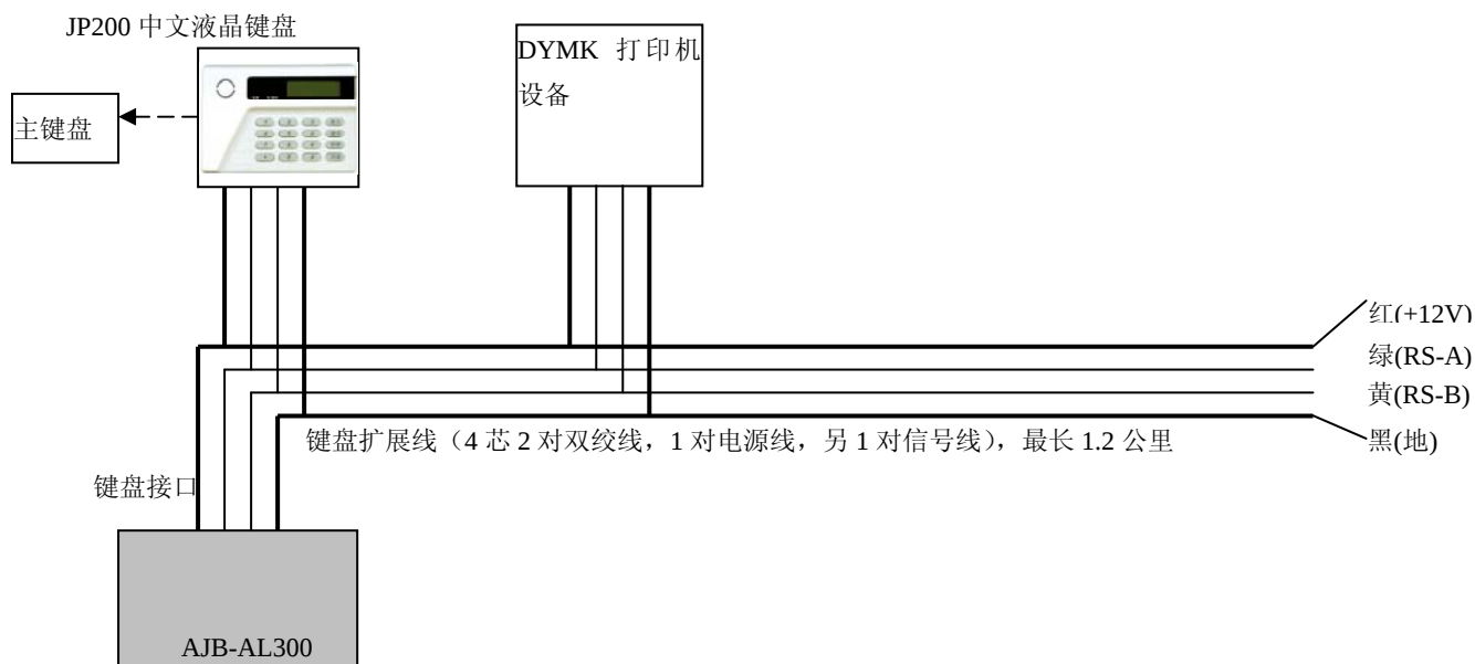
AJB-AL300 与主键盘、打印设备连接示意图
