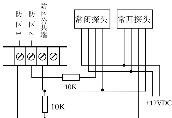
探测设备接线示意图
