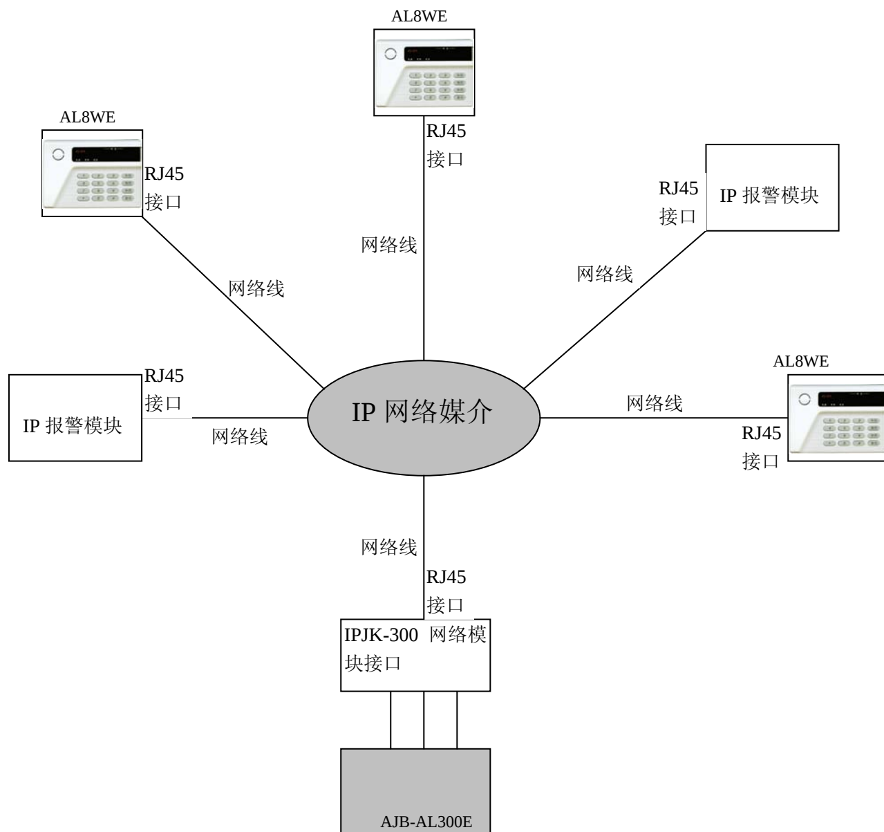
AJB-AL300V20 与网络接警设备连接示意
