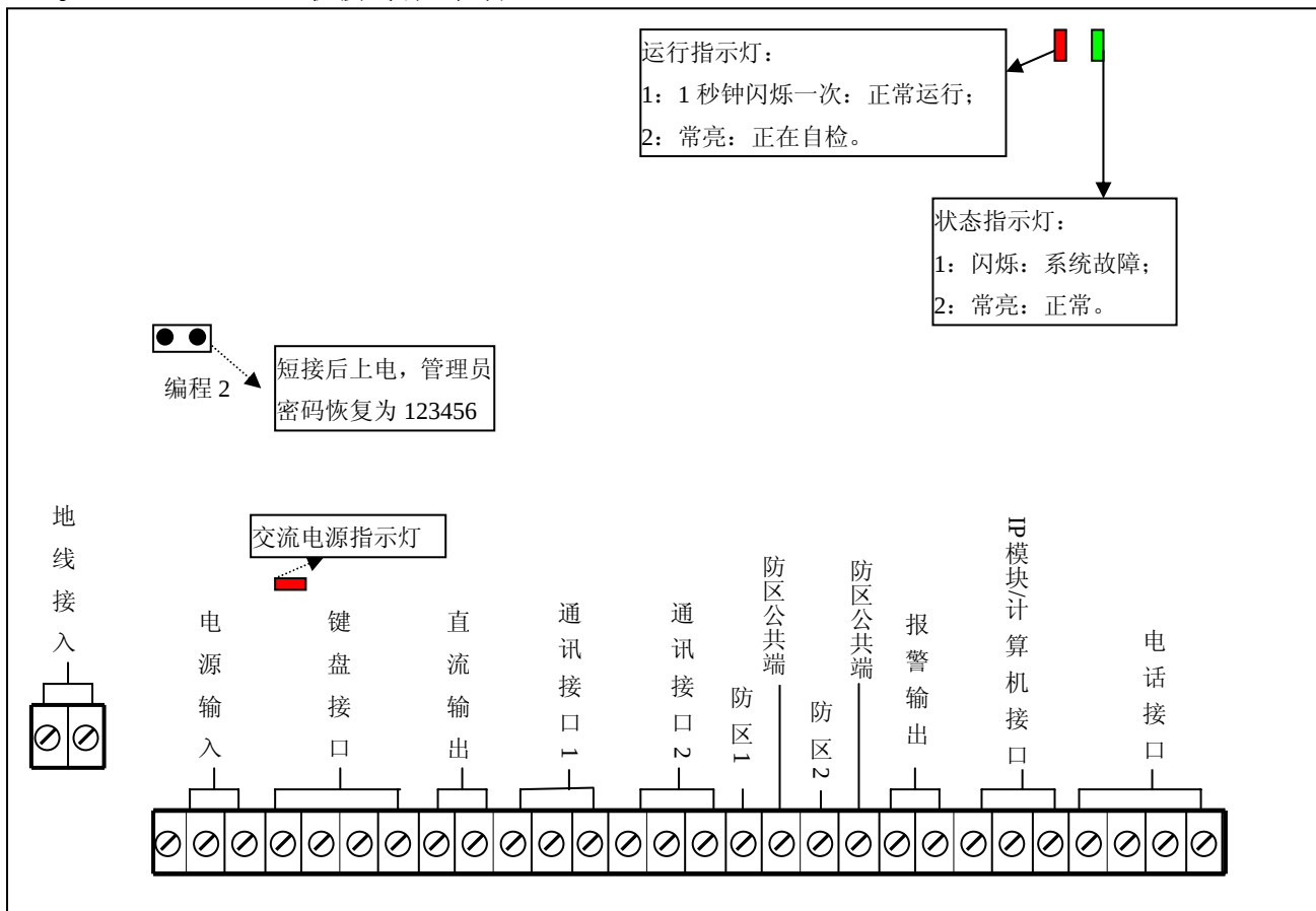
AJB-AL300V3.0 报警主机端口示意图
