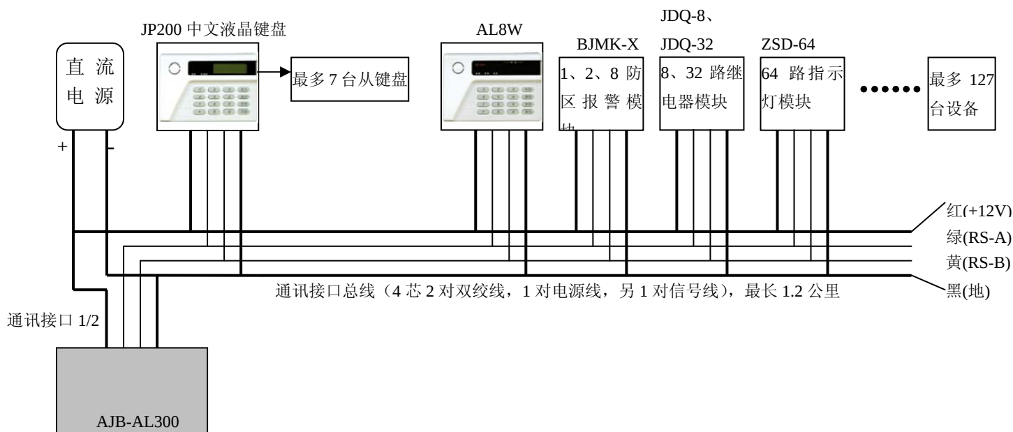
AJB-AL300 与总线设备连接示意图
