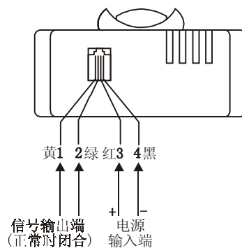
液化气探测器接线示意图
