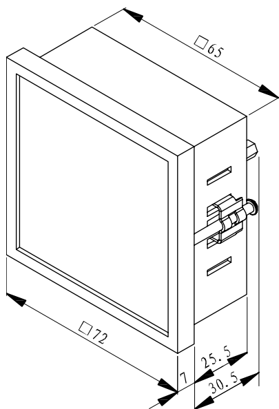
PD194Z-3XYS 表头显示部分
