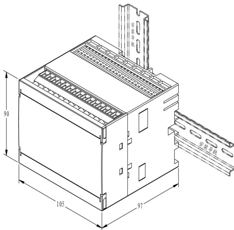
JD194-BS4Z8 尺寸及安装 (PD194Z-3XYS 主体相同):
