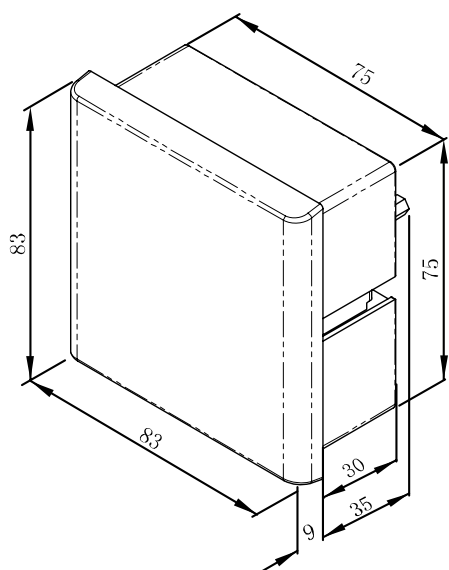
PD194Z-3XYS 表头显示部分
