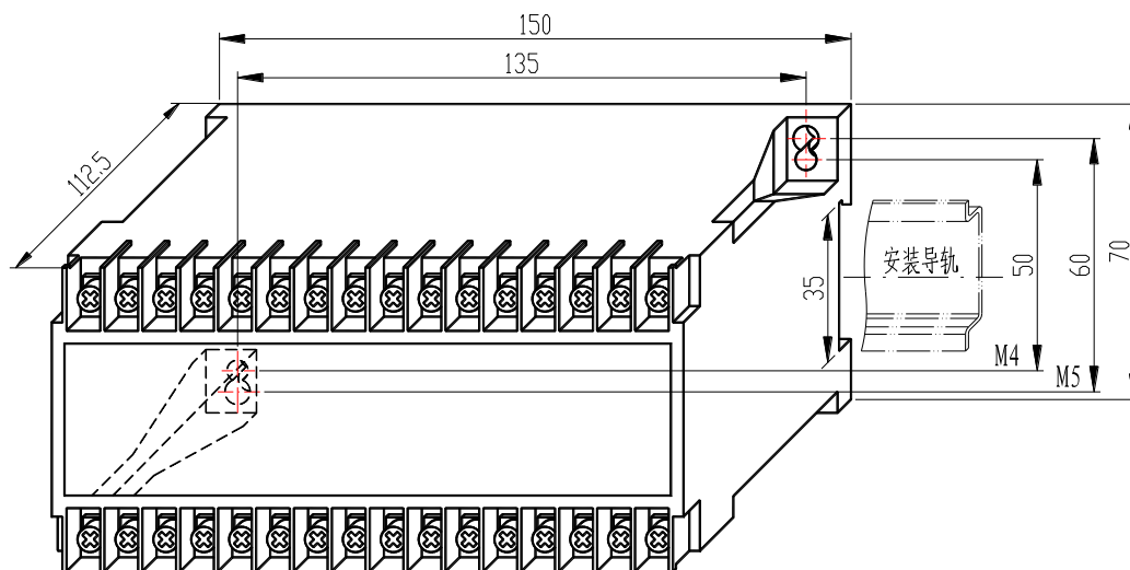
JD194-BS4Z8 尺寸及安装 (PD194Z-3XYS 主体相同):
