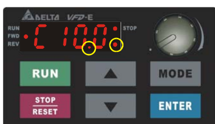
显示 10000~65535 时，只会显示前 3 个字符，另外小数点第一位的灯会亮著且右下方 LED 灯会亮起，表示显示值乘以 100 倍，如图中所显示的值表示为 10000~10099
