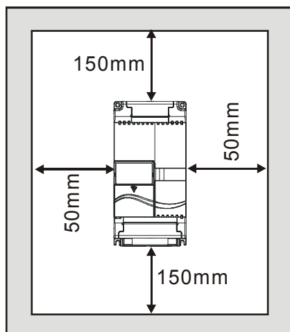
单机设置图
