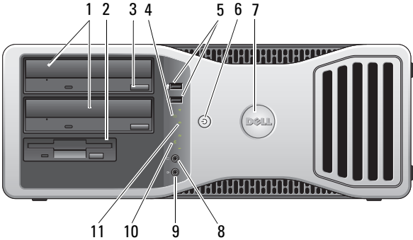
台式计算机 — 正面视图
