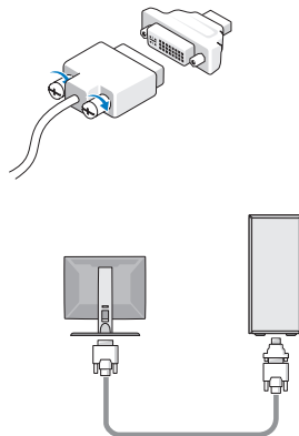
f 连接至 DVI 适配器的 DisplayPort
