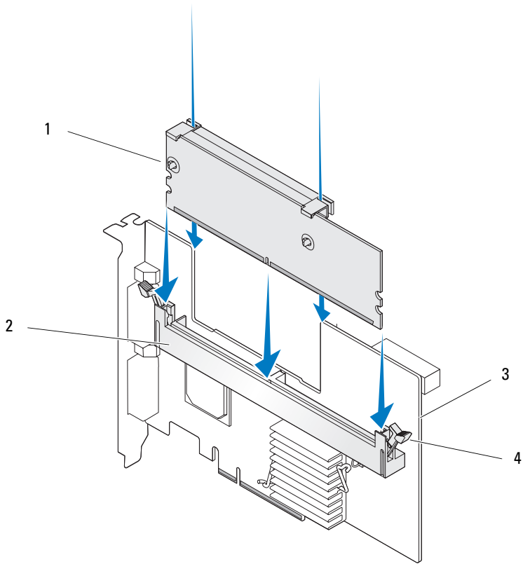
그림 4. DIMM (Dual In-line Memory Module) 설치
