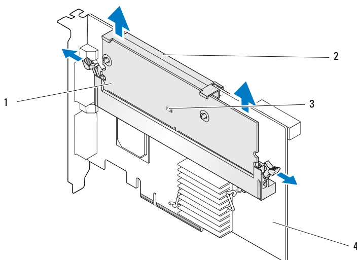
図 1 PERC xE アダプタのダーティーキャッシュ LED の位置
