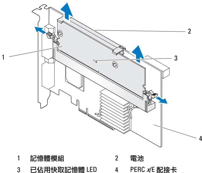
圖 1. PERC x/E 配接卡已佔用快取記憶體 LED 位置
