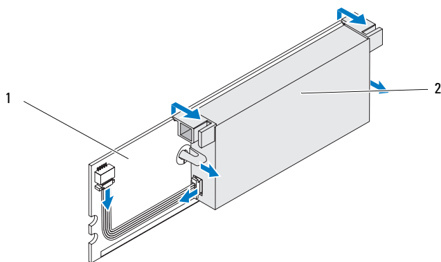
図 2 BBU の取り外し
