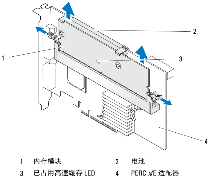
图 1. PERC x/E 适配器已占用高速缓存 LED 位置
