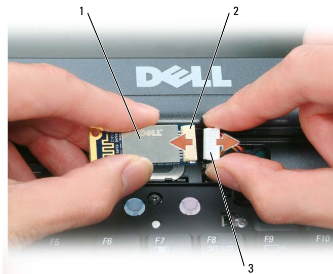
1 插卡
