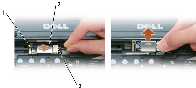
1 金属卡舌
