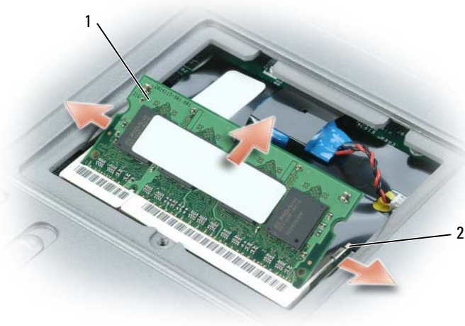
1 内存模块
