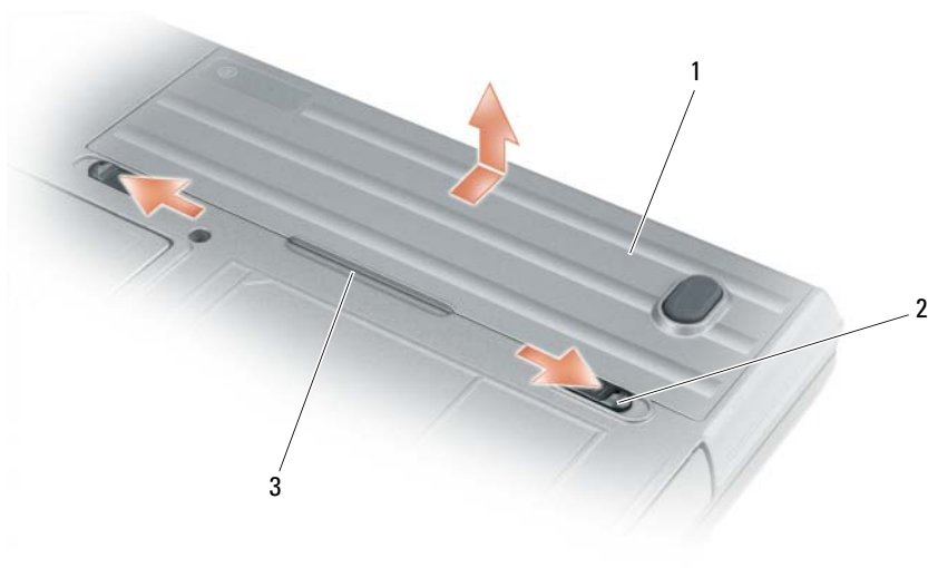
1 電池 2 電池凹槽釋放門鎖 (2) 3 電池彈片
