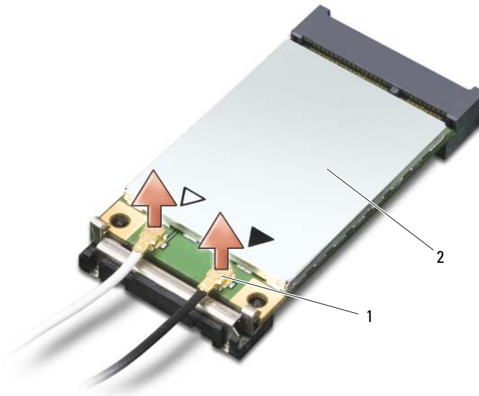
1 天線纜線連接器 (2) 2 WLAN 卡
