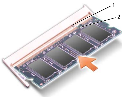
1 卡舌 2 槽口
