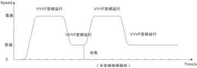
图 7-9 全变频驱动 快慢循环节能曲线图
