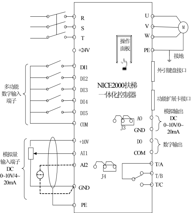
图 3-3 适应于 NICE-E(1)-A-4013 ~ NICE-E(1)-A-4060 控制器
