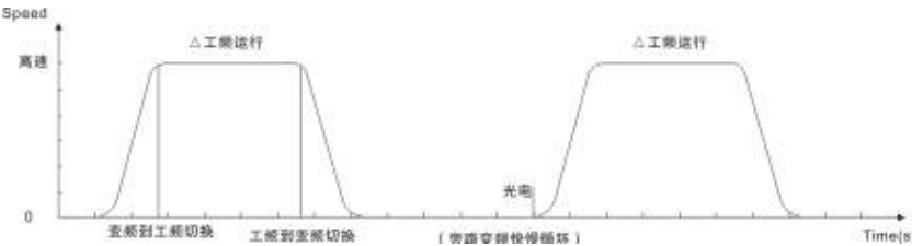
图 7-6 旁路变频驱动 快停循环节能曲线图
