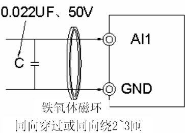
图 3-6 模拟量输入信号处理接线图
