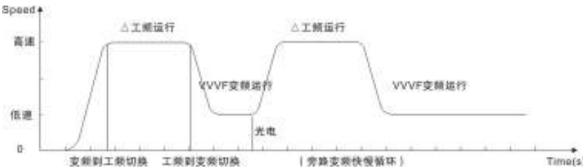
图 7-4 旁路变频驱动 快慢循环节能曲线图
