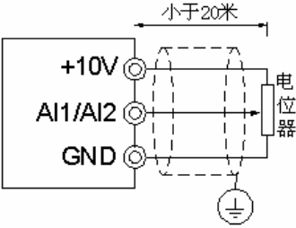
图 3-5 模拟量输入端子接线示意图
