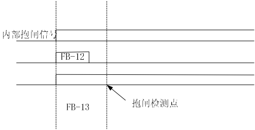
图 6-3 抱闸输出时序图
