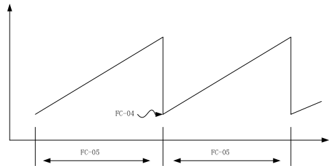
图 6-5 同步信号周期
