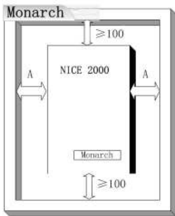
图 3-1 安装位置
