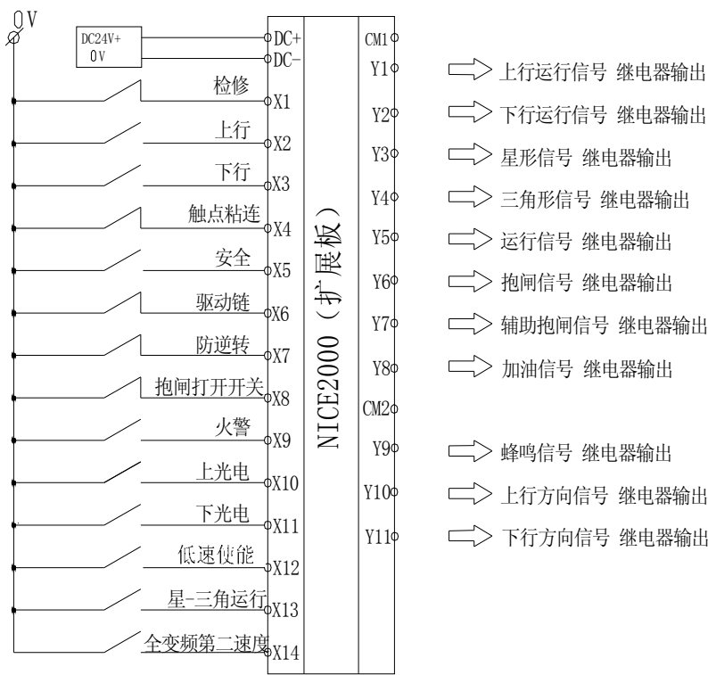
图 3-4 适应于 NICE-E(1)-A-4013 ~ NICE-E(1)-A-4060 扩展板
