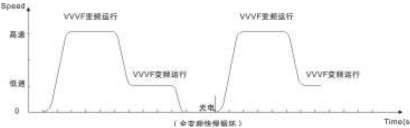
图7-10 全变频驱动 快慢停循环节能曲线图
