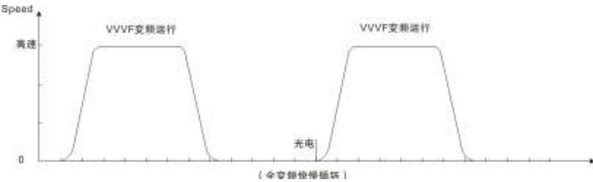
图 7-11 全变频驱动 快停循环节能曲线图
