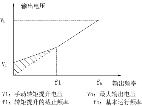
图6-1 手动转矩提升示意图
