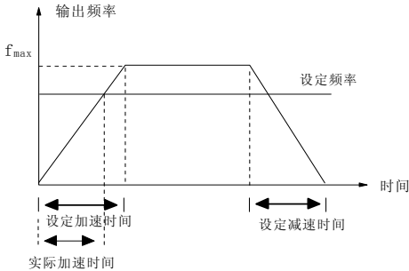
图6-2 加减速时间示意图
