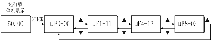
图4-7 快捷菜单的调出
