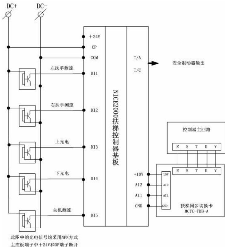
图 7-3 NICE2000 基板接线（包含同步切换卡）
