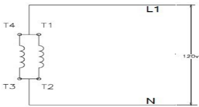
单相---单相的连接
