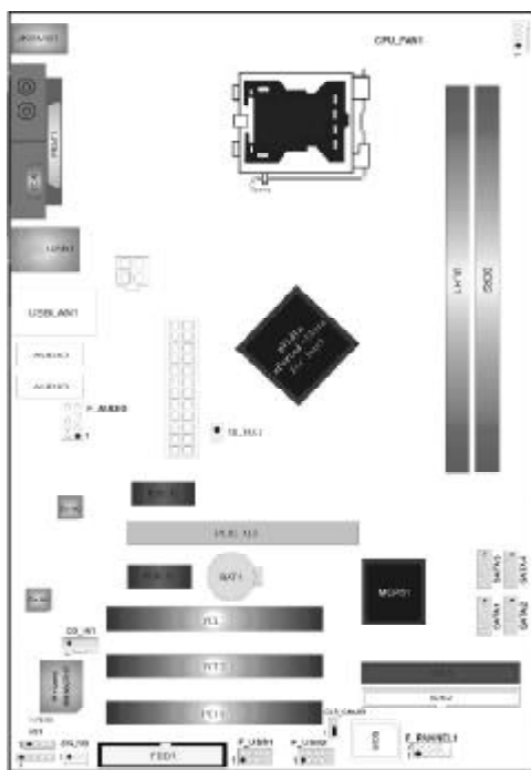
主机板布局图
