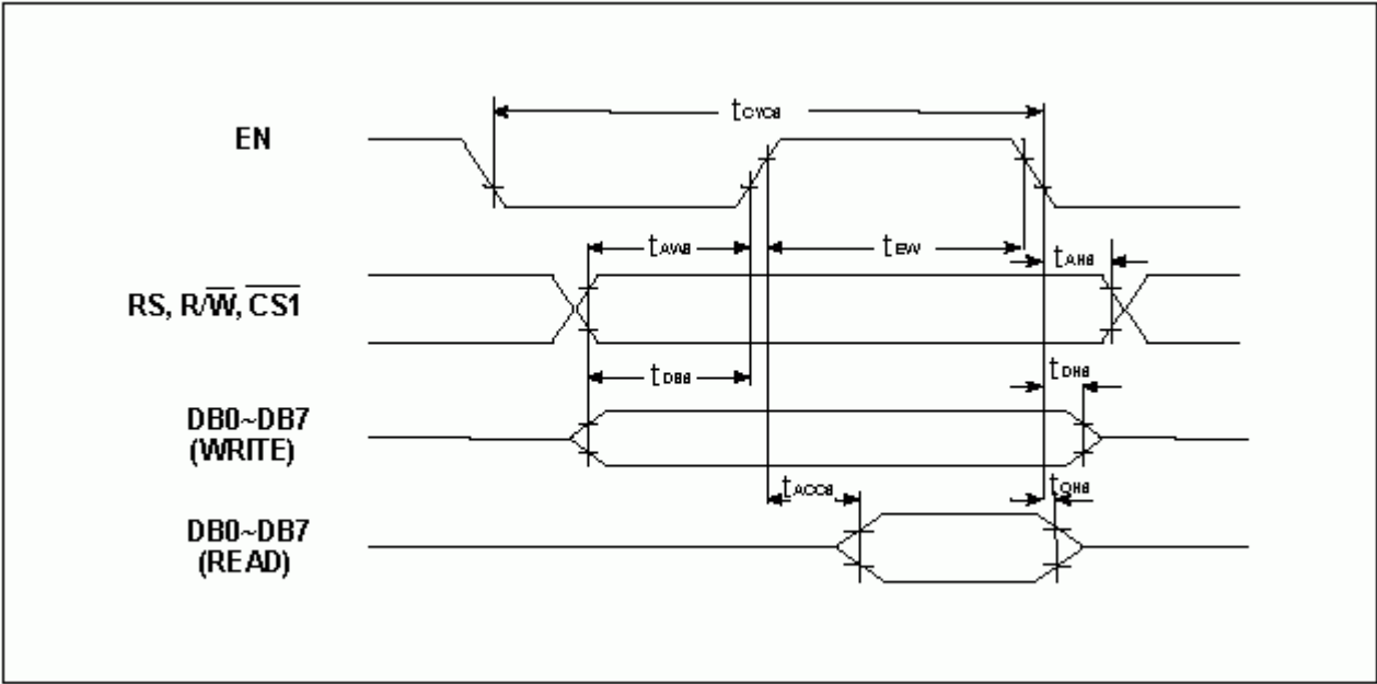
图3-4: 8-bit 6800 MCU 对CM160128-3暂存器/Data进行读取/写入动作
