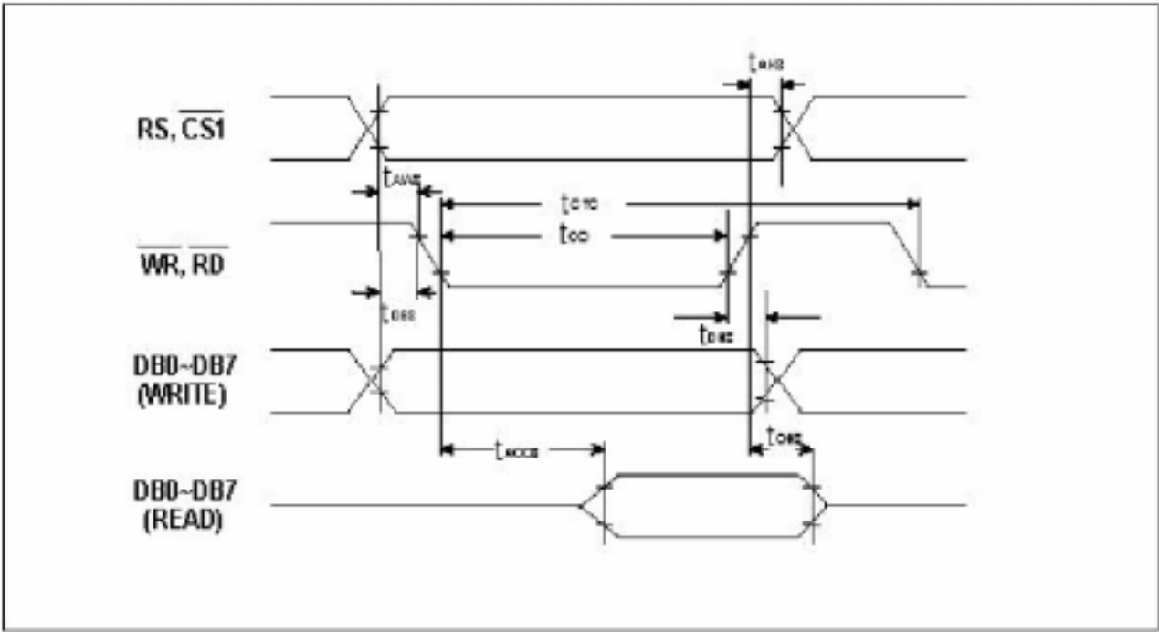
图3-2 8B1t8080MCU对寄存器/DATA进行读取/写入动作
