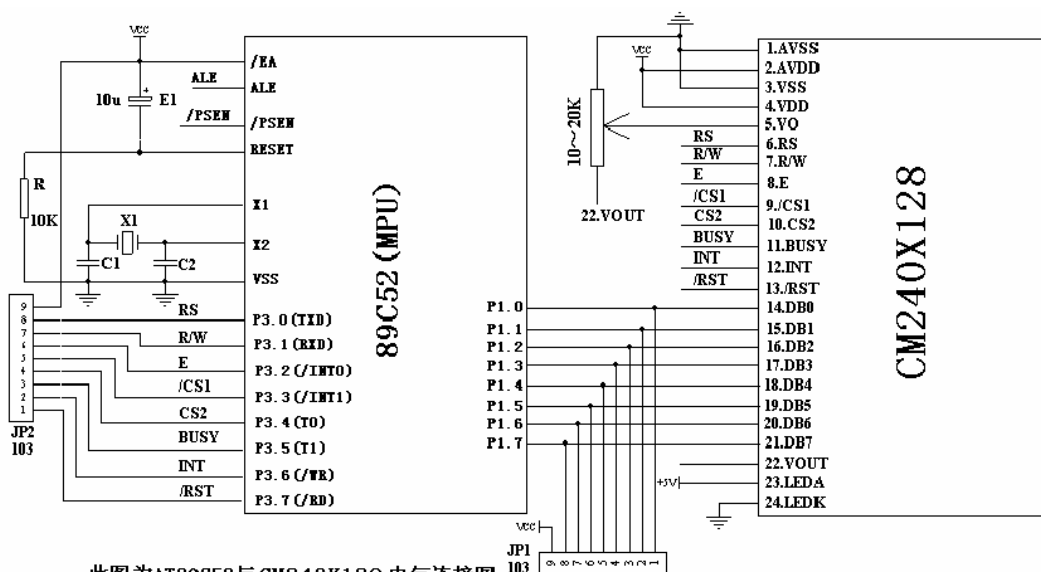
此图为AT89C52与CM240X128 电气连接图
