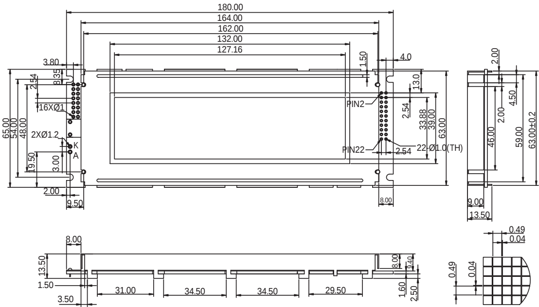
CM15X4模块尺寸图
