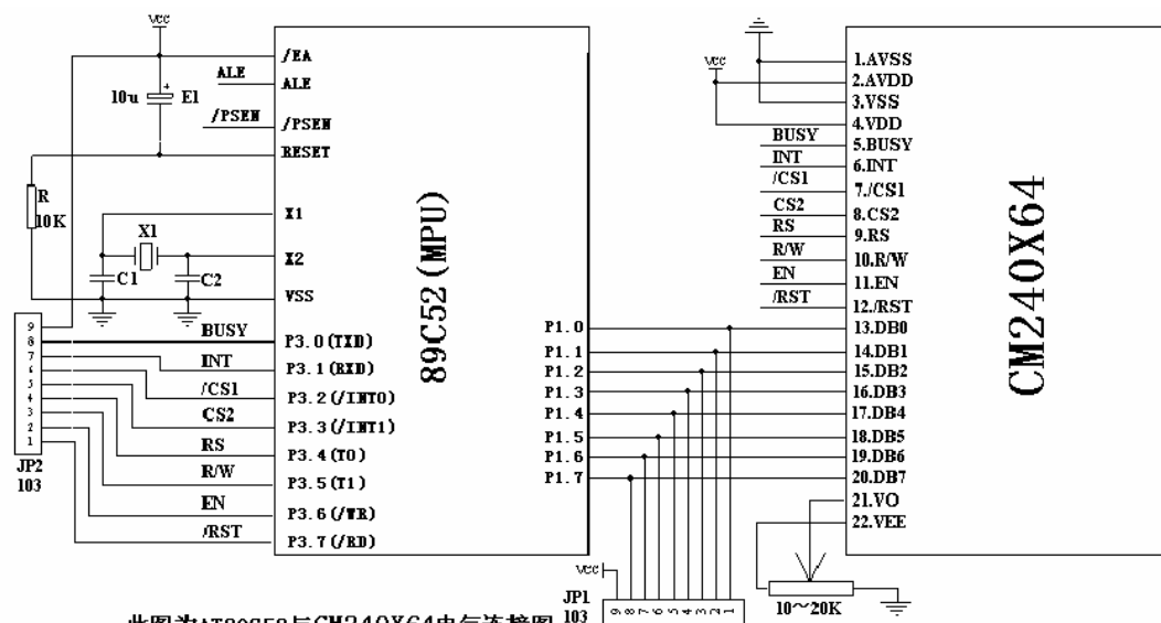
此图为AT89C52与CM240X64电气连接图
