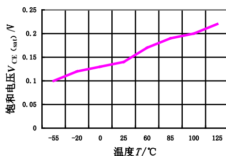
集-发饱和电压 V_{\text{CE(sat)}} 随温度 T 变化的曲线
