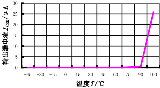
输出漏电流 I_{\text{CBO}} 随温度 T 变化的曲线
