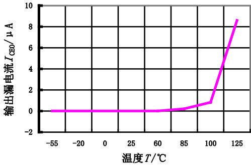
输出漏电流 I_{\text{CE0}} 随温度 T 变化的曲线
