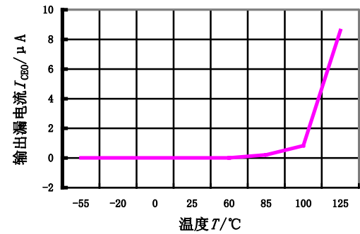
输出漏电流 I_{CBO} 随温度 T 变化的曲线
