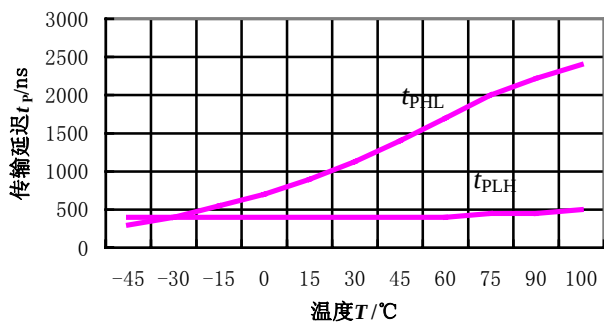
传输延迟 t_p 随温度 T 变化的曲线
