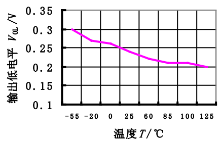
输出低电平 V_{OL} 随温度 T 变化的曲线
