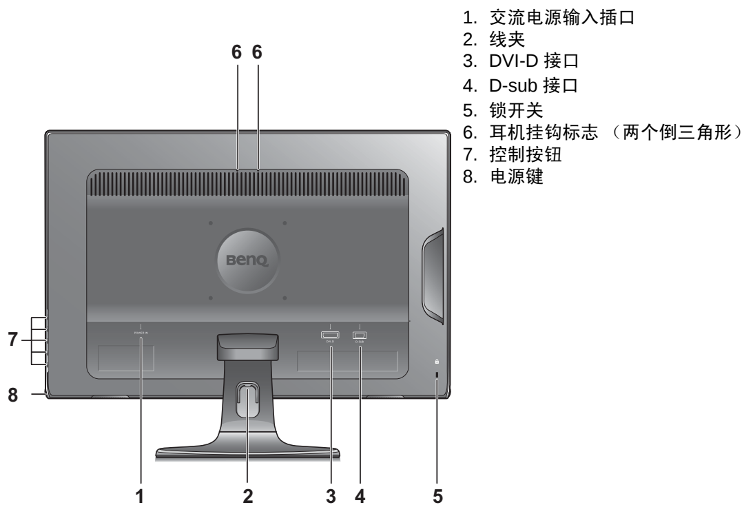
后视图
