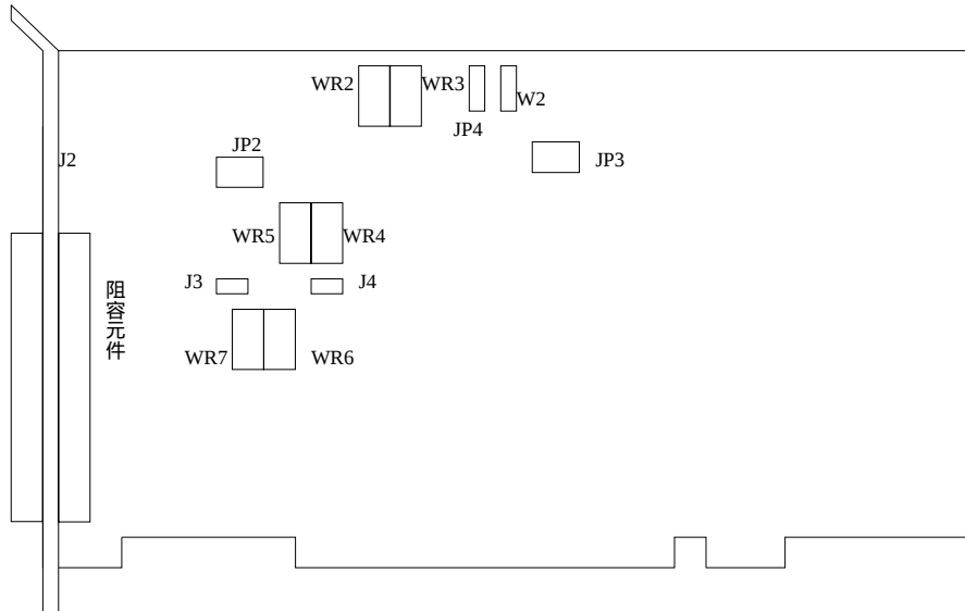
图 3 操作元件布置
