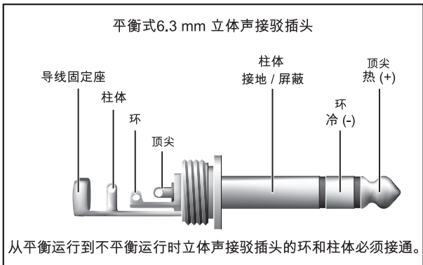
图 8.1 : 6.3mm 立体声道接驳插头
