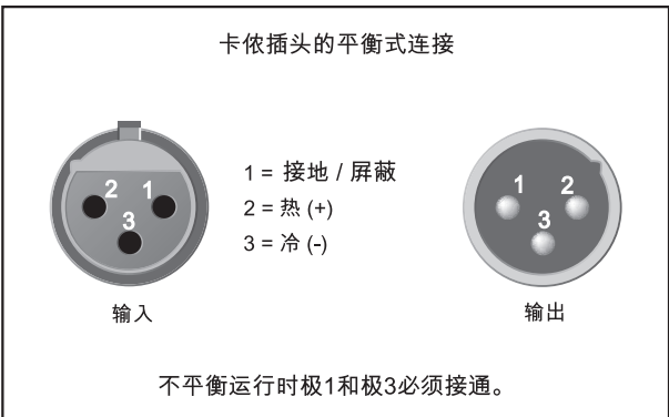
图 8.2 : XLR 插头
