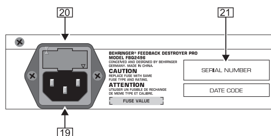
图 3.4: 电源连接、保险丝座和产品序号
