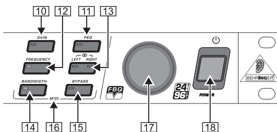
图 3.3: FBQ2496 右侧的操作元件
