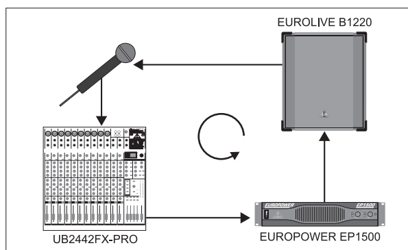
图 2.1：反馈回路的产生
