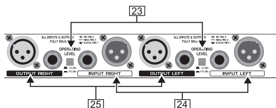
图 3.6: FBQ2496 背面的接口
