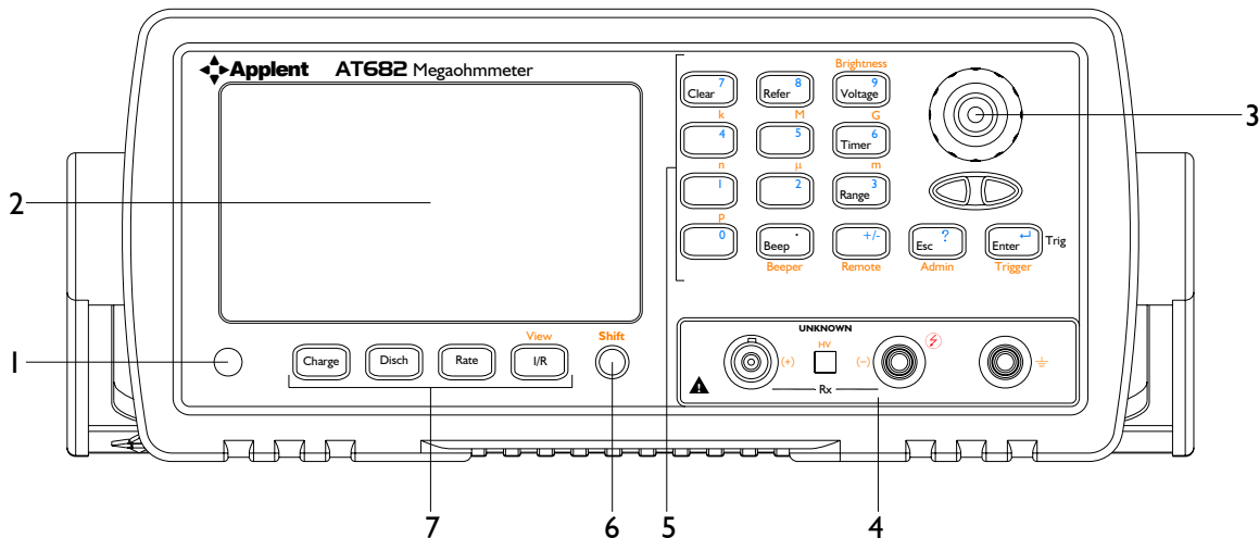
图 3-1 前面板
