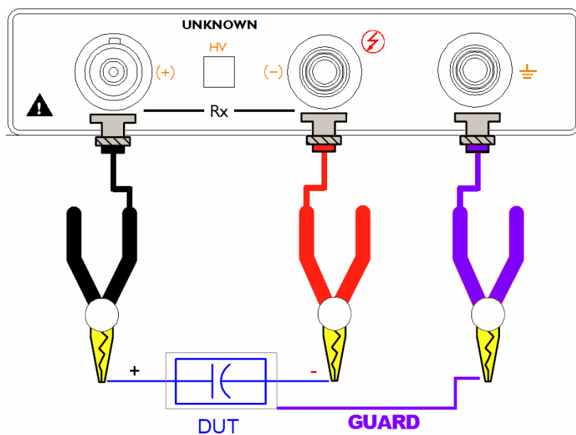
图 3-7 测试端
