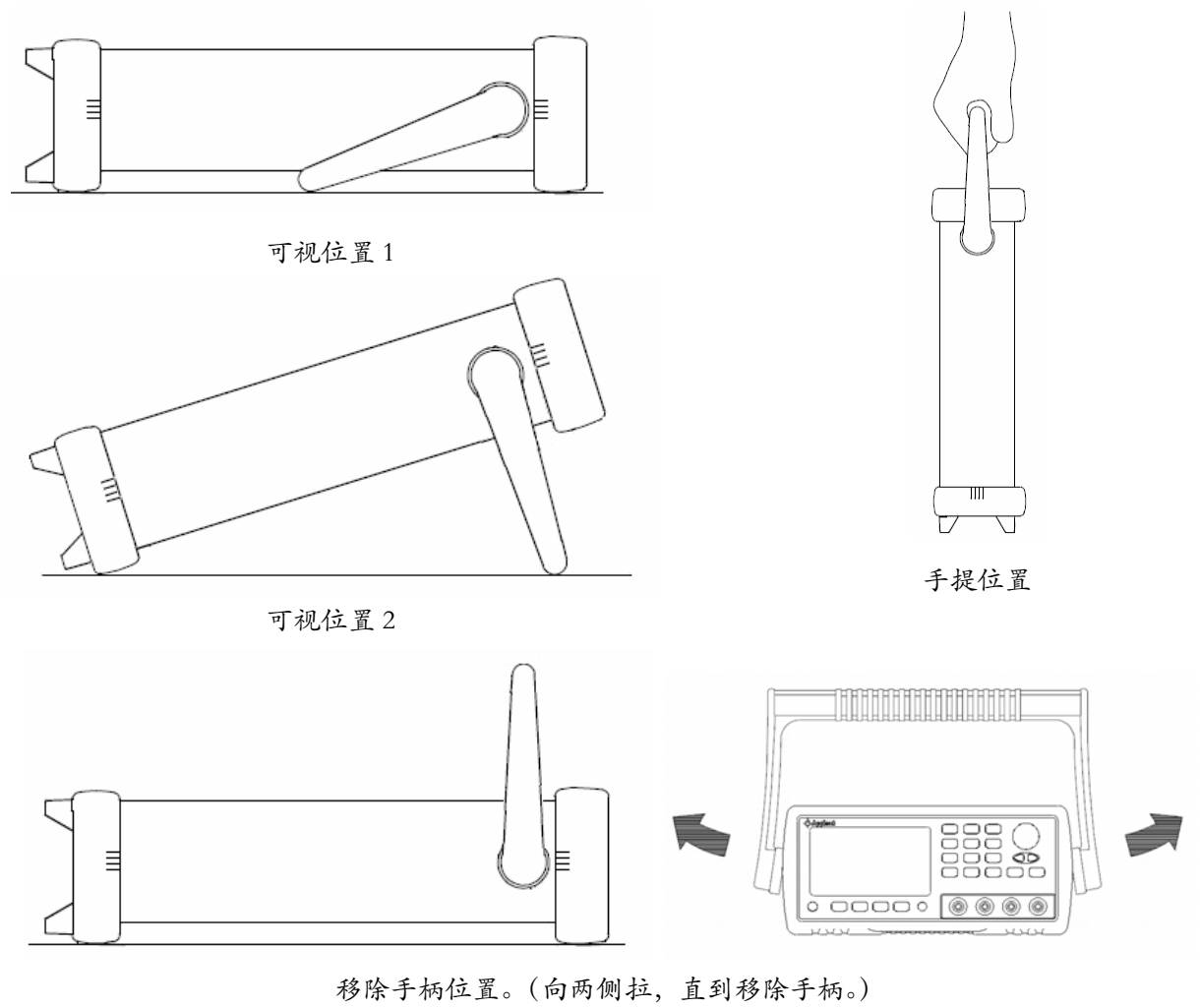
图 3-6 仪器手柄
