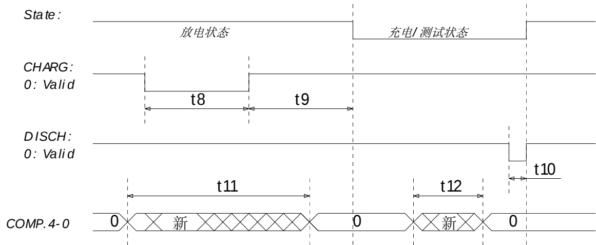
图 5-4 周期表
