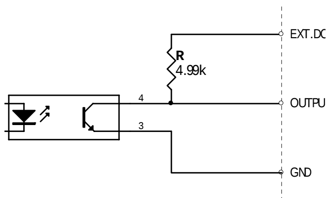
图 5-2 内部原理图
