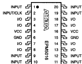
SOIC
