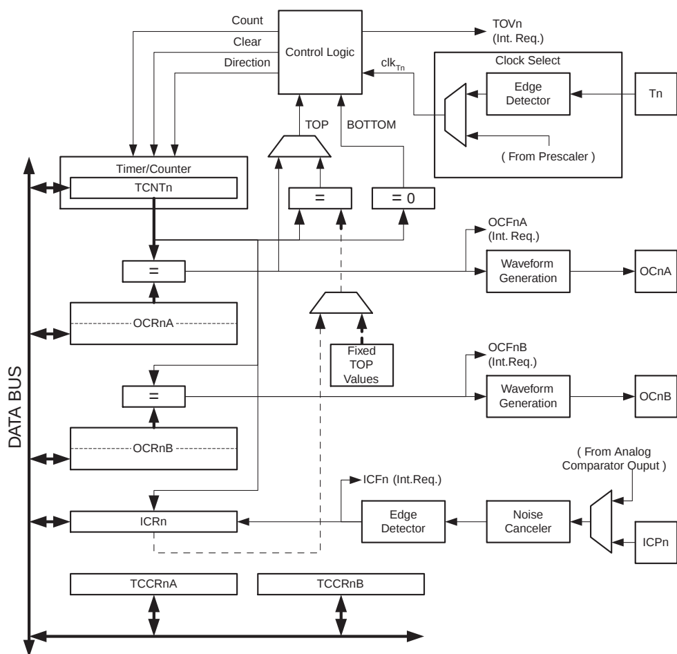
Figure 32. 16 位 T/C 框图 (1)
