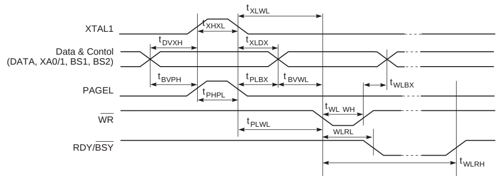
Figure 110. 并行编程时序，有时序要求的加载序列 (1)
