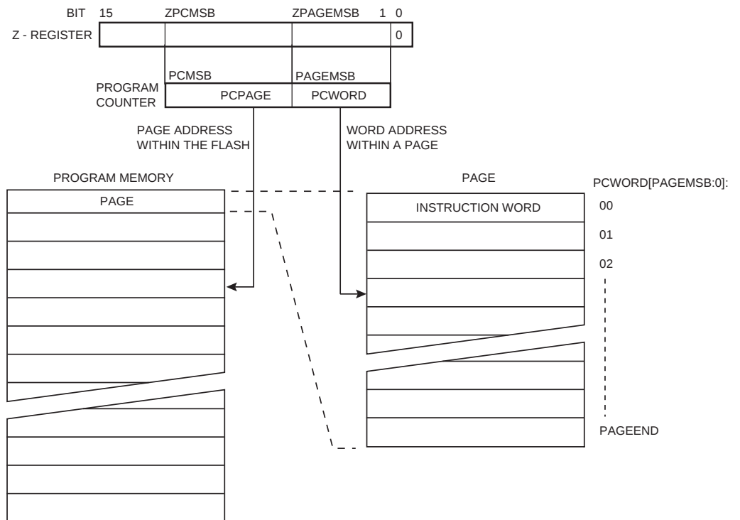
Figure 103. SPM 的寻址 (1)
