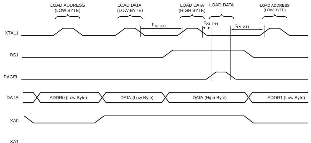
Figure 110. 并行编程时序，有时序要求的加载序列 (1)
