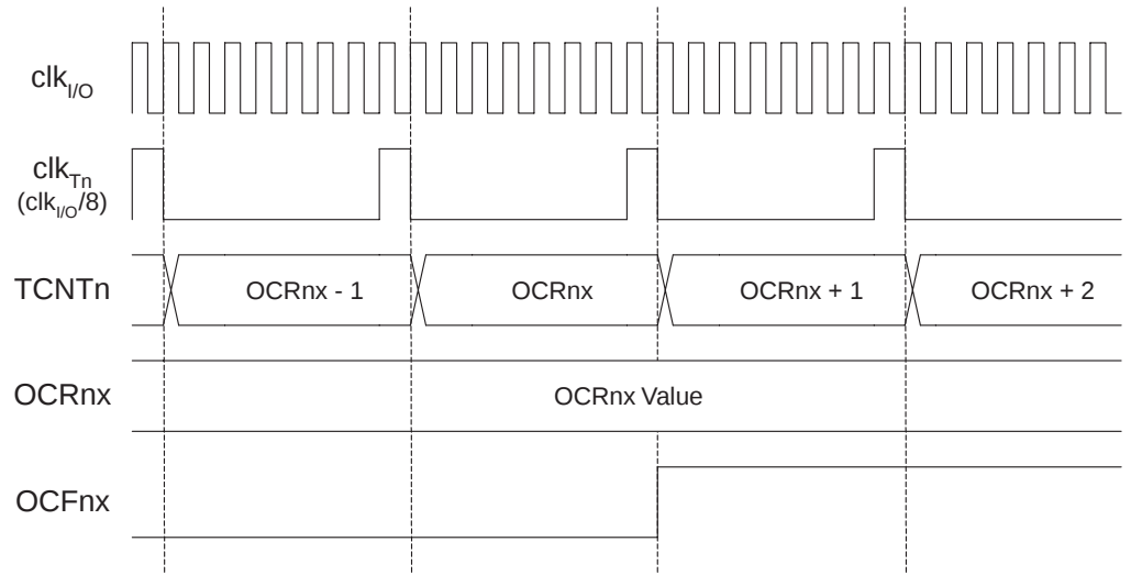
Figure 42. T/C 时序图，置位 OCF1x，预分频器为 f_{clk\_I/O}/8
