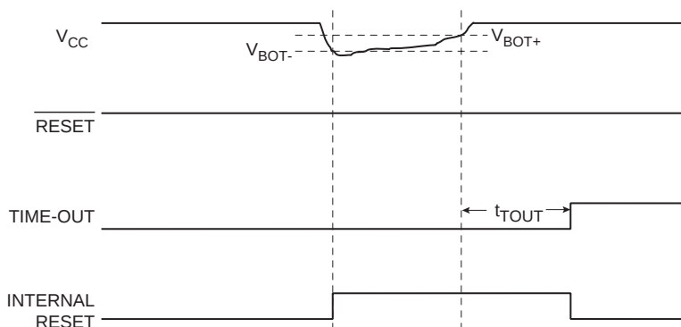
Figure 18. 工作过程中发生掉电检测复位
