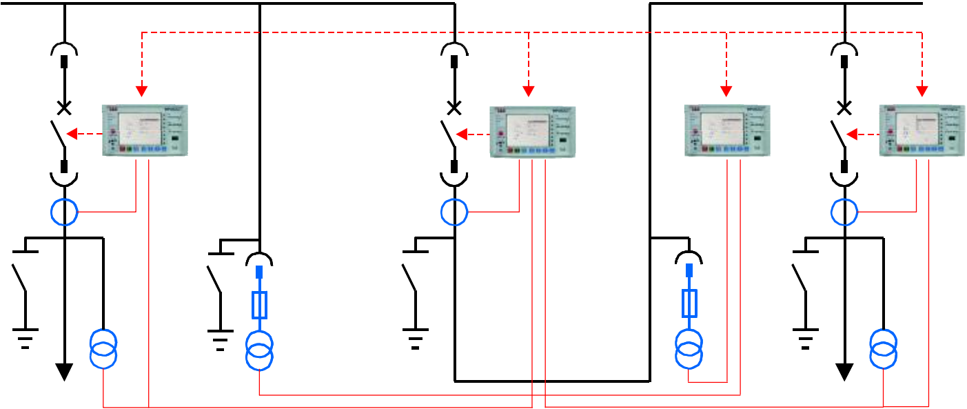
带 REF542plus 的 UniGear ZS1 开关设备单线图。具有自动或手动切换及保护测量功能。
