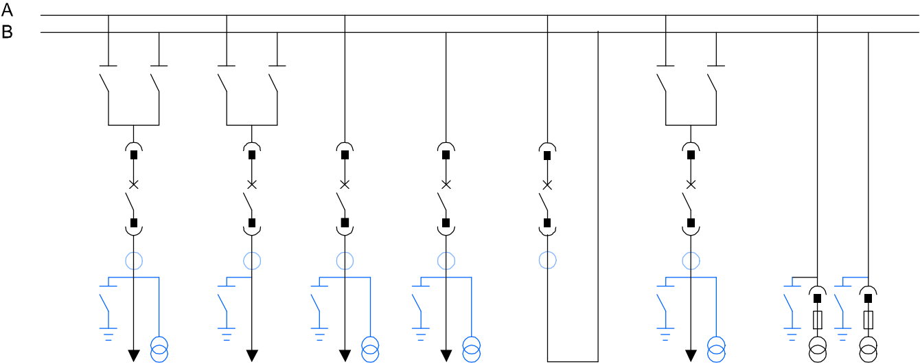
带母联开关的双母线系统
