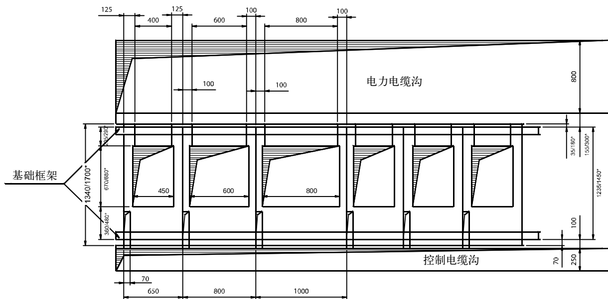
图17.3 配电室电缆沟道典型布置图
