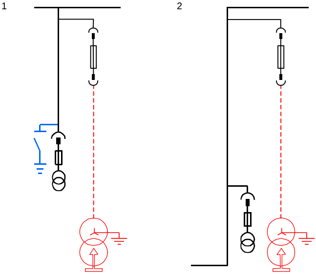
1 M-带接地变压器的PT 单元 | 2 RLM-带 PT 和接地变压器的母线提升单元
