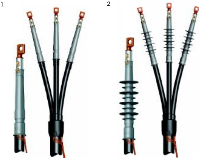
1 SOT单芯和三芯户内终端 | 2 SOT单芯和三芯户外终端
