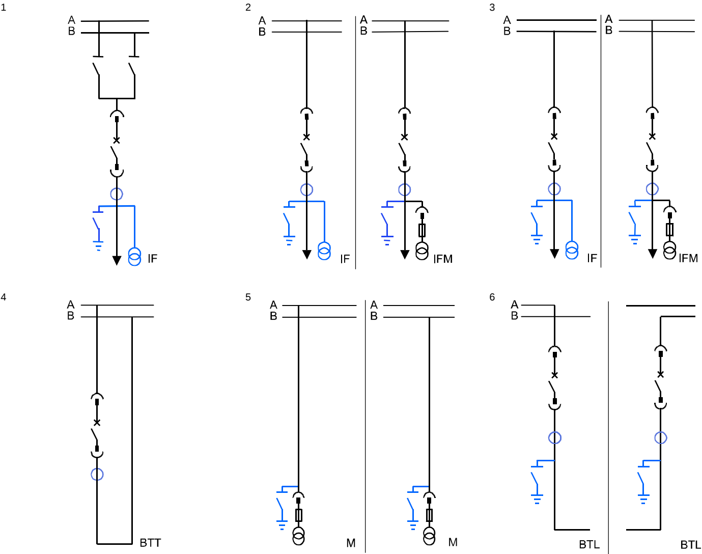
典型方案的单线图
