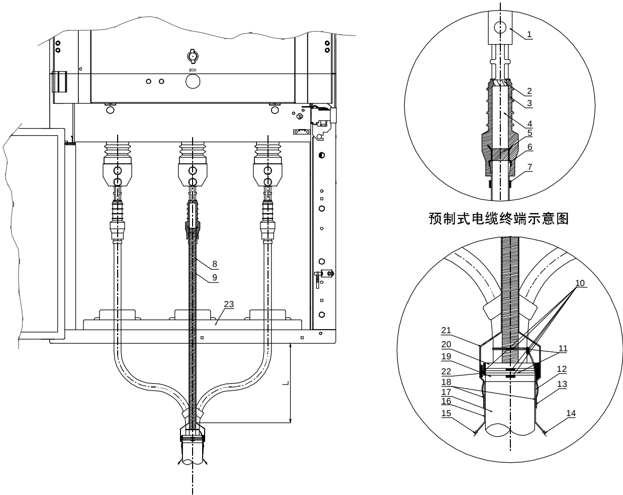
图17.5 电缆连接示意图
