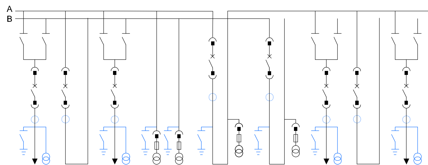
双母线分断系统
