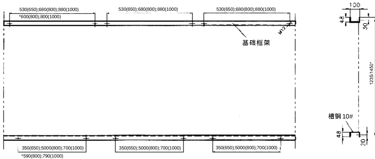
图 17.4 柜宽为 1000,800,650mm 三种柜型的基础框架典型加工图, 其中 24kV 柜宽为 600,800mm 两种。
