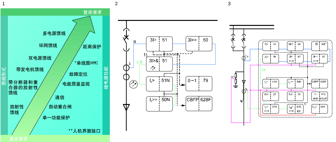
1 基本要求和复杂要求馈线的比较 | 2 典型基本要求馈线 | 3 典型复杂要求馈线
