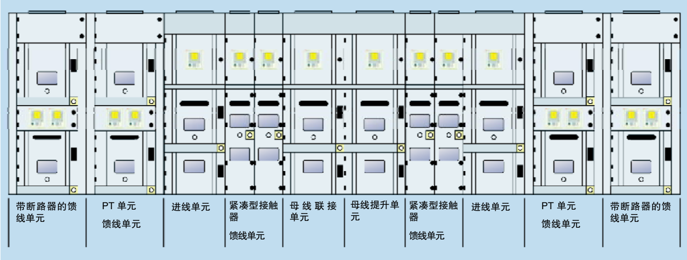
UniGear ZS1 单母线柜，双层柜和 UniGear ZVC 的组合方案
