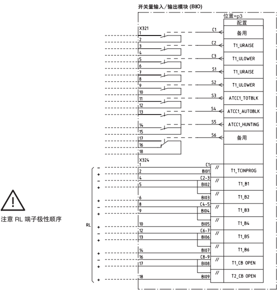
图 34. 开关量输入/输出 (BIO) 选项 (端子 X321 和 X324)
