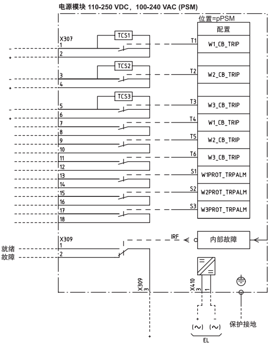
图 25. 电源模块 (PSM)，交流，110-250V，直流
