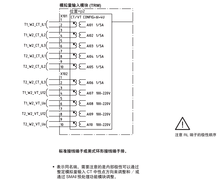
图 33. 模拟量输入模块 (TRM)
