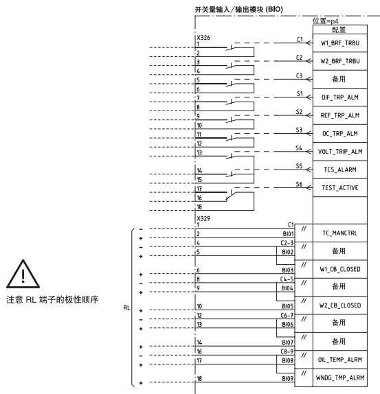
图 22. 开关量输入/输出 (BIO) 选项 (端子 X326 和 X329)
