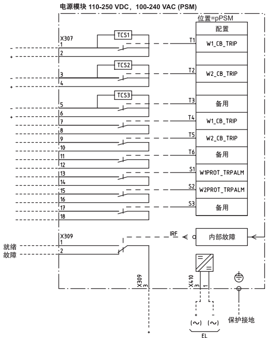
图 19. 电源模块 (PSM), 交流, 110-250V, 直流
