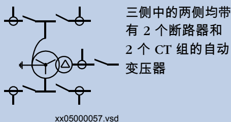
图 4. 差动保护和其他保护的 CT 组排列
