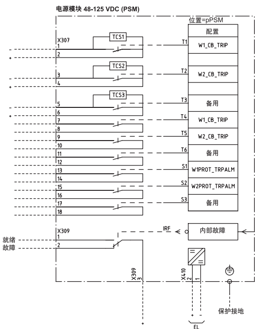
图 18. 电源模块 (PSM) 48-125V, 直流
