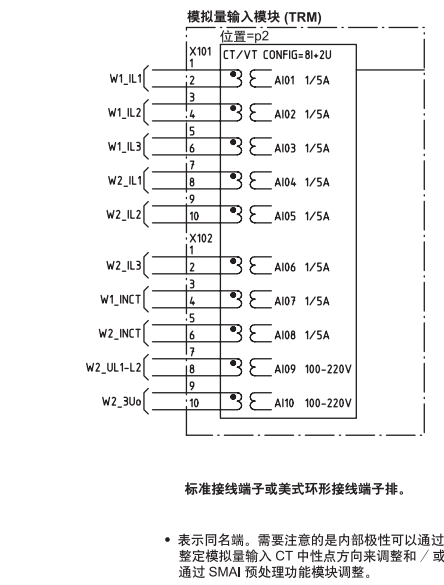
图 20. 模拟量输入模块 (TRM)
