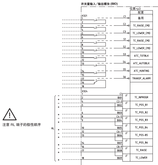
图 21. 开关量输入/输出 (BIO) 选项 (端子 X321 和 X324)
