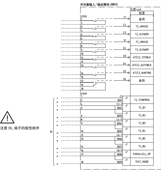
图 35. 开关量输入/输出 (BIO) 选项 (端子 X326 和 X329)
