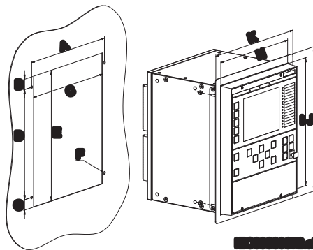
图 8. 将装置嵌入式安装于面板开孔上。
