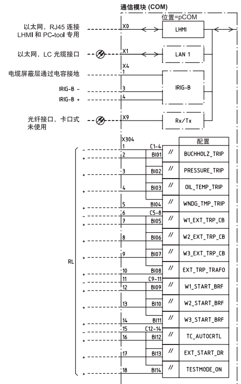
图 23. 通讯模块 (COM)
