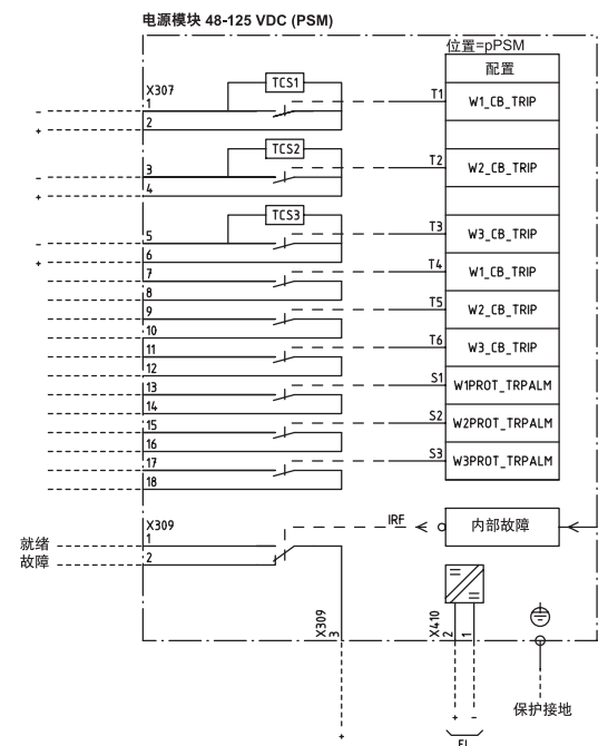
图 24. 电源模块 (PSM) 48-125V, 直流
