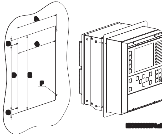
图 10. 将装置半嵌入式安装于面板开孔上
