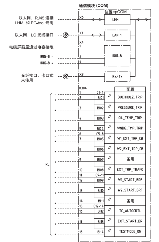
图 17. 通讯模块 (COM)
