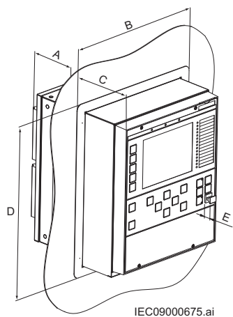
图 11. 半嵌入式安装
