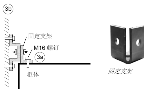
用固定支架和橡胶垫从上方固定柜体 ( 侧视图 )
