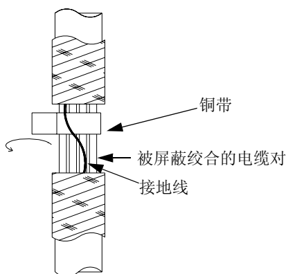
屏蔽层的导电面被翻露出来
