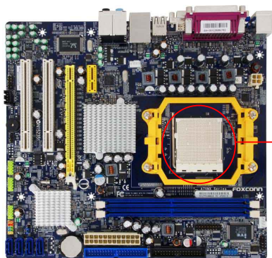
插座针脚1对应的边角
