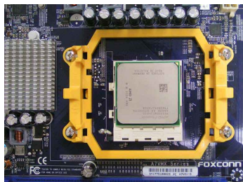
2. 将CPU的金三角标记对准插座上的针脚1位置, 然后将其轻放入插座中。
