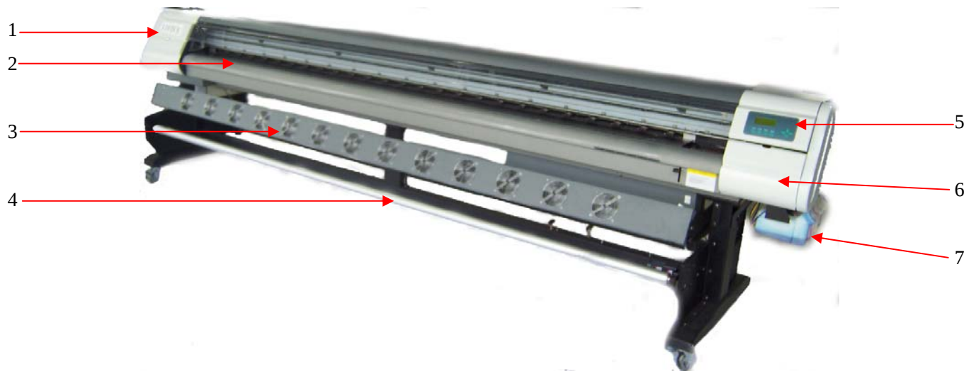
图 4-1 33VBX 机器视图
