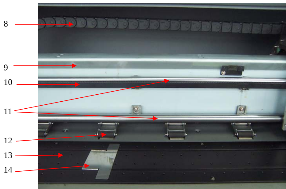
图 4-2 机械组件
