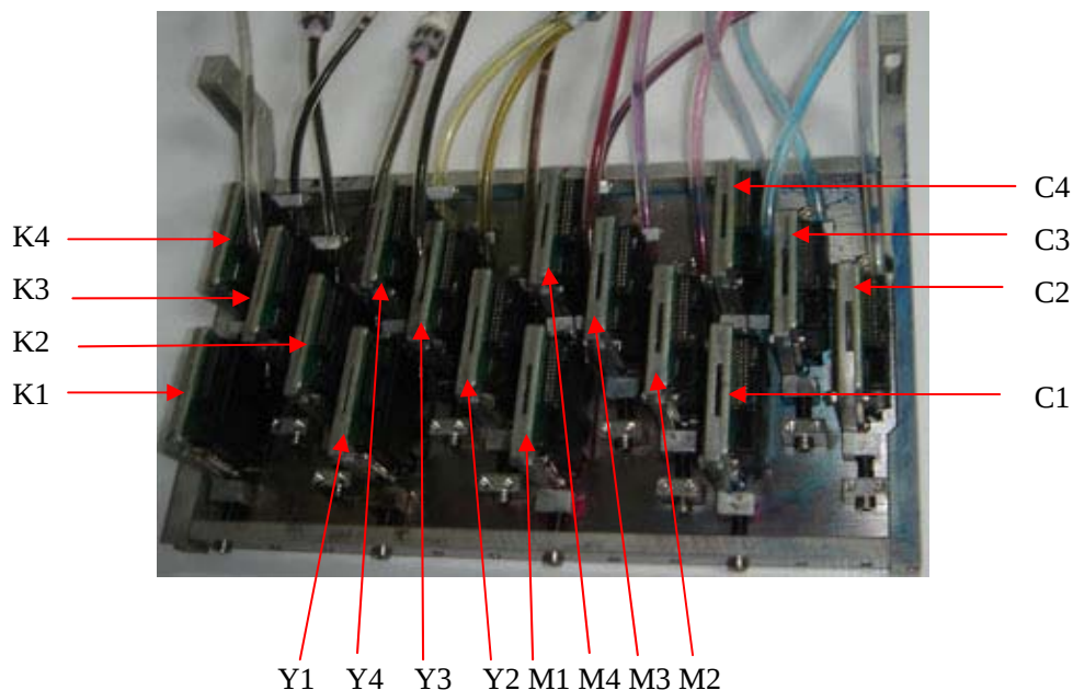
图 3-2 喷头转接板连线安插顺序
