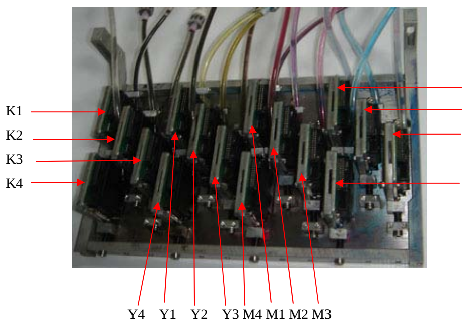
图 11-6 喷头排列
