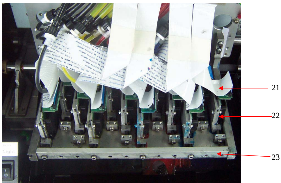
图 4-5 喷头
