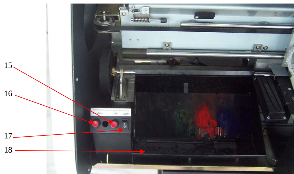
图 4-3 清洗装置
