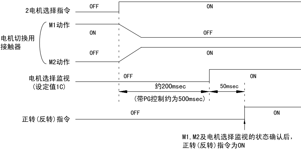
图 7.37 电机 1 → 电机 2 切换运行场合的时序图
