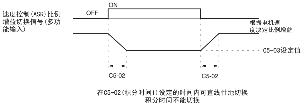
图 6.16 速度控制 ASR 比例增益切换
