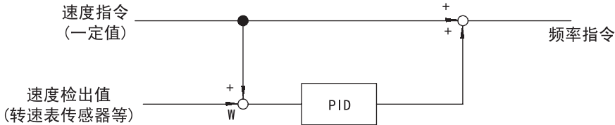
图 7.25 设定值 3、4 的应用举例
