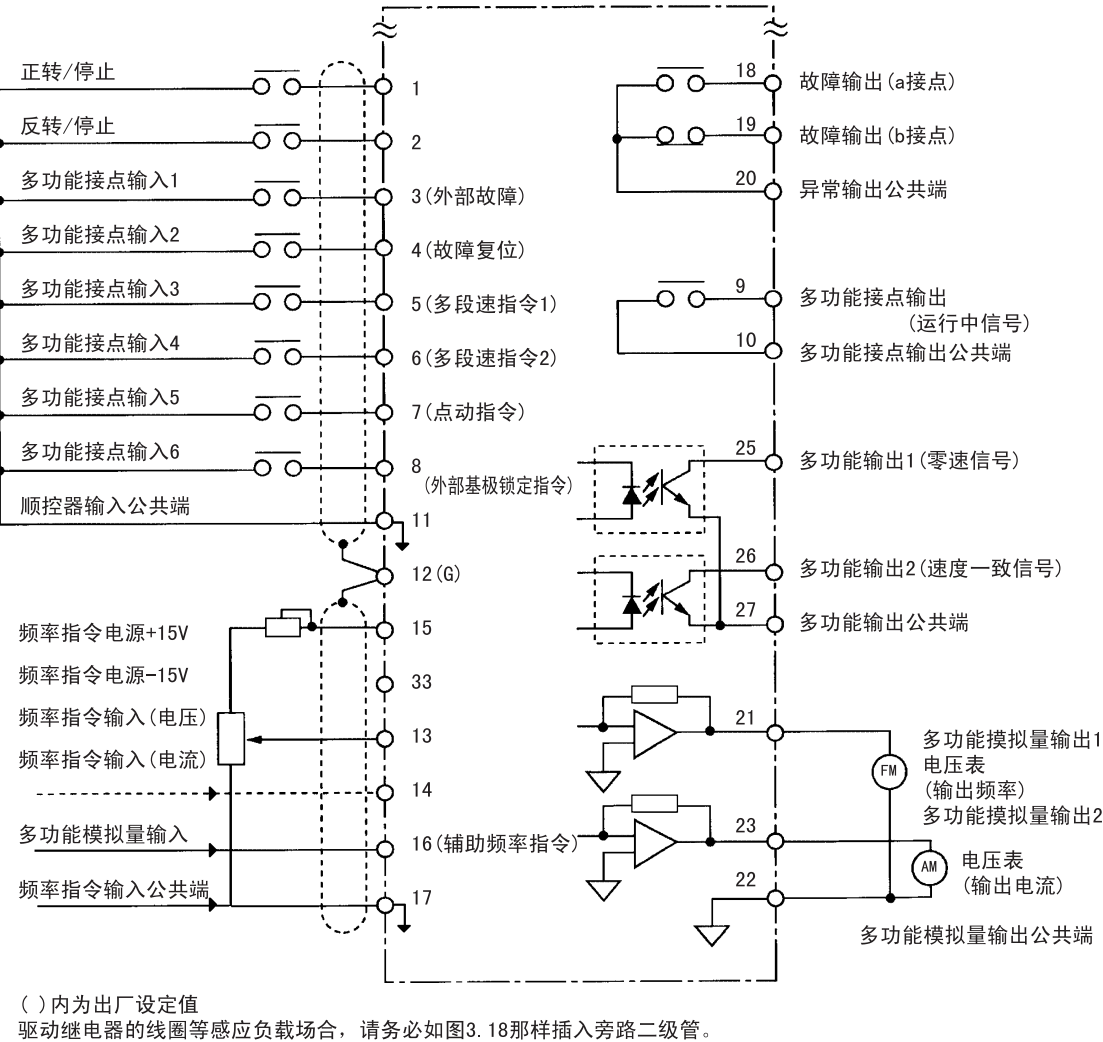
图 3. 20 控制回路端子的连接
