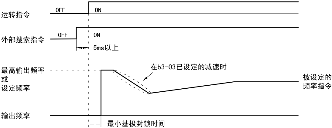
图 7.42 外部搜索指令的时序图
