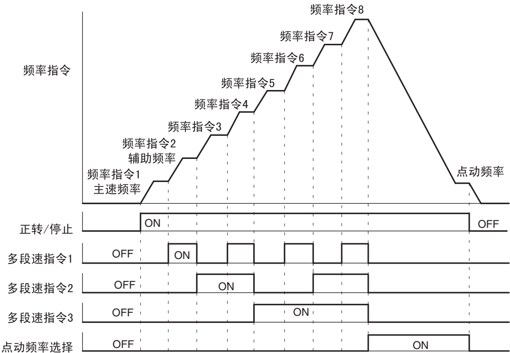
图 6.10 多段速指令 / 点动频率选择的时序图
