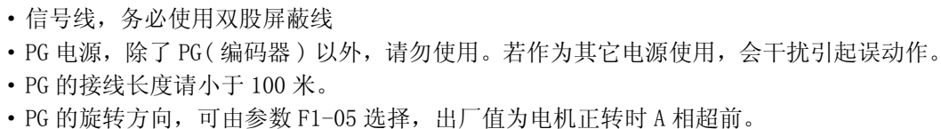
图 3.29 PG-X2 卡的接线
