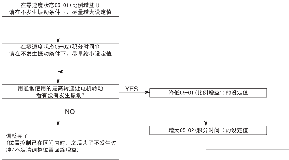
图 6.17 增益的调整顺序
