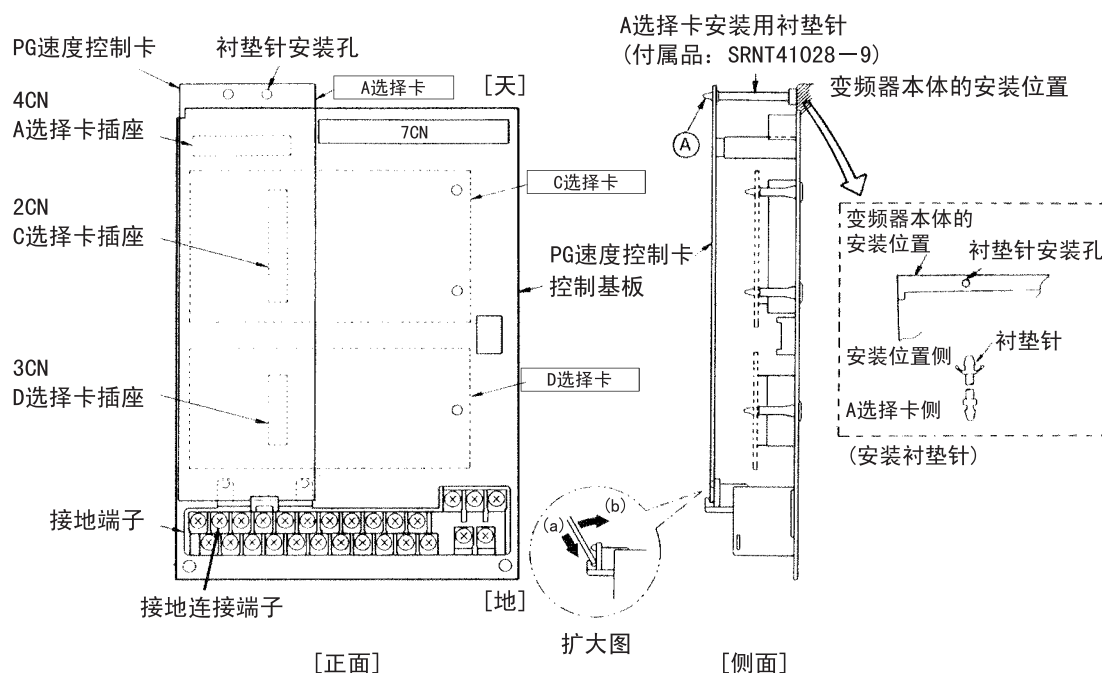
图 3.22 PG 速度控制卡的安装
