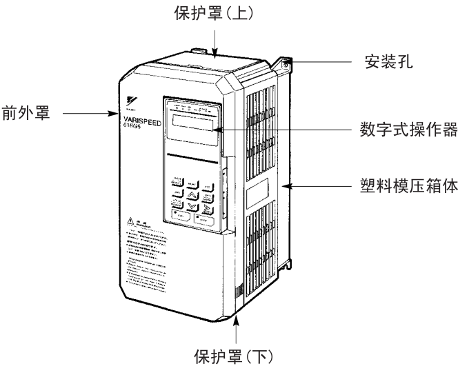
图 1.2 VS-616G5 的外观，以 CIMR-G5A20P4 形 (200V 0.4kW) 为例。 卸掉前外罩状态的 200V 级 0.4kW 变频器如图 1.3 所示。
