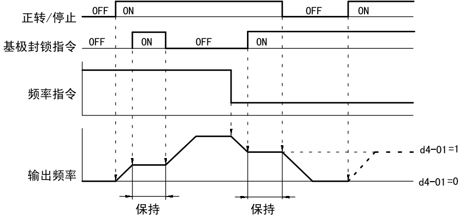
图 7.3.5 加减速停止
