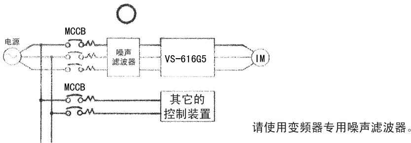
图 3.8 电源侧噪声滤波器的正确设置举例
