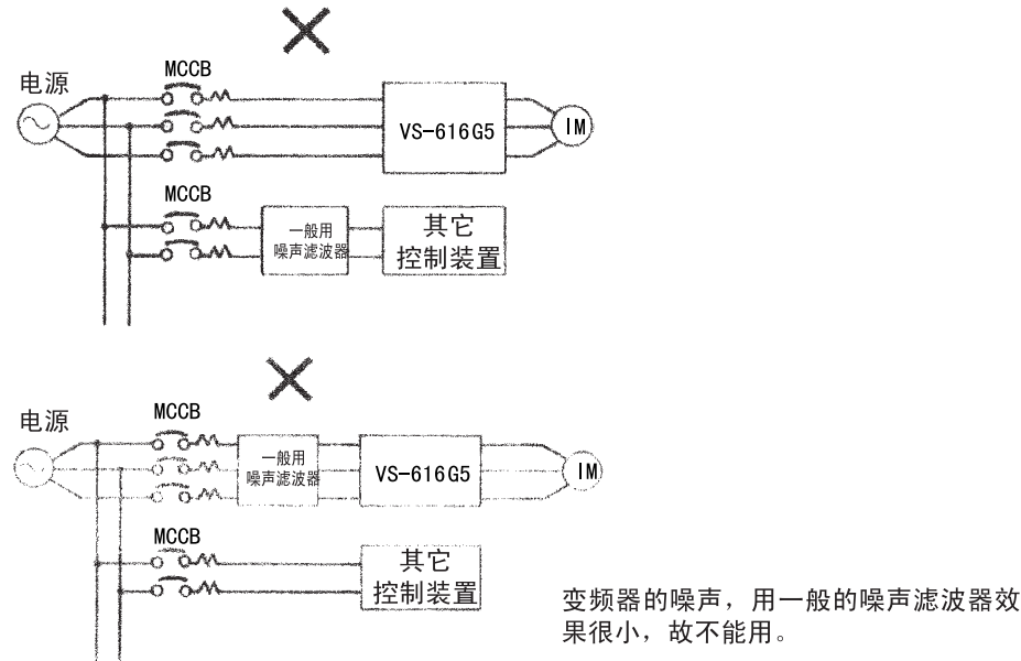
图 3.9 电源侧噪声滤波器的不正确设置举例
