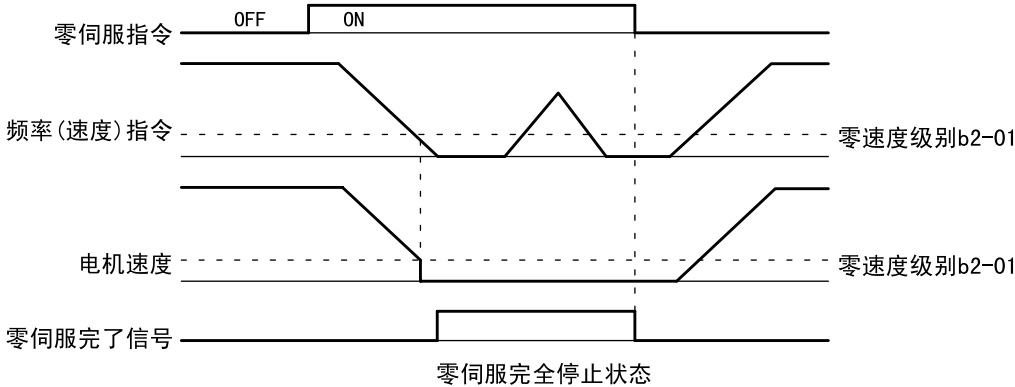
图 7.8 零伺服时序
