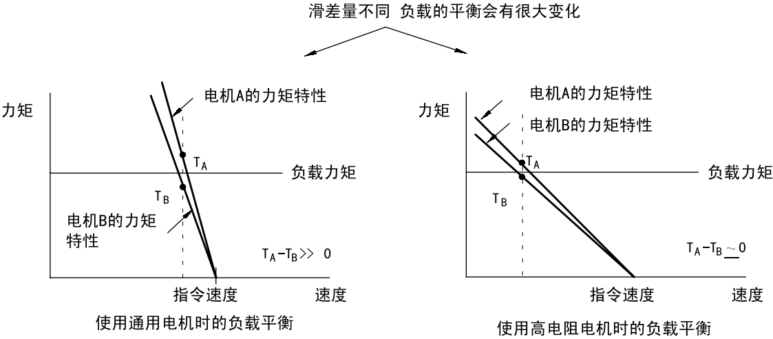
图 7.6 DR00P 下降控制功能
