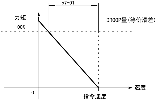
图 7.7 DR00P 下降控制增益
