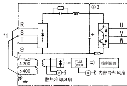
CIMR-G5A4055~4160形 (55~160kW)
