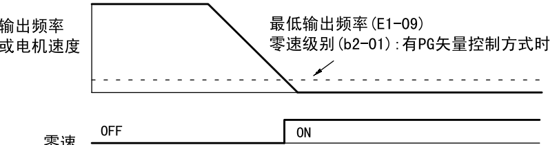
图 7.44 零速的时序图
