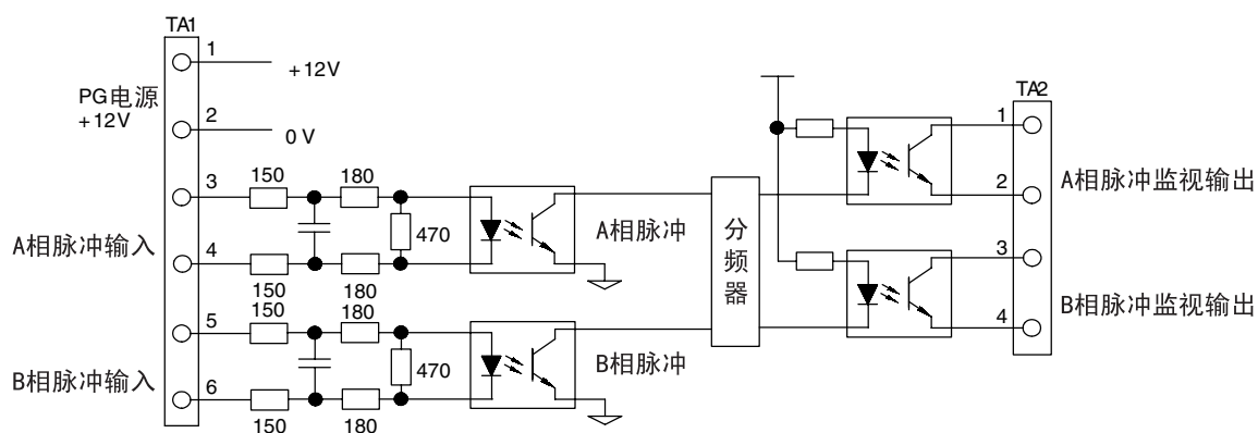
图 3.26 PG-B2 的接线
