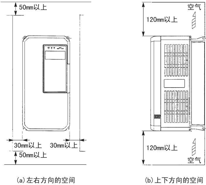
图 2.1 VS-616G5 的安装方向和空间
