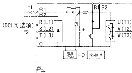
CIMR-G5A40P4~41P5形 (0.4~1.5kW)
