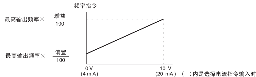
图6.2 增益与偏置
