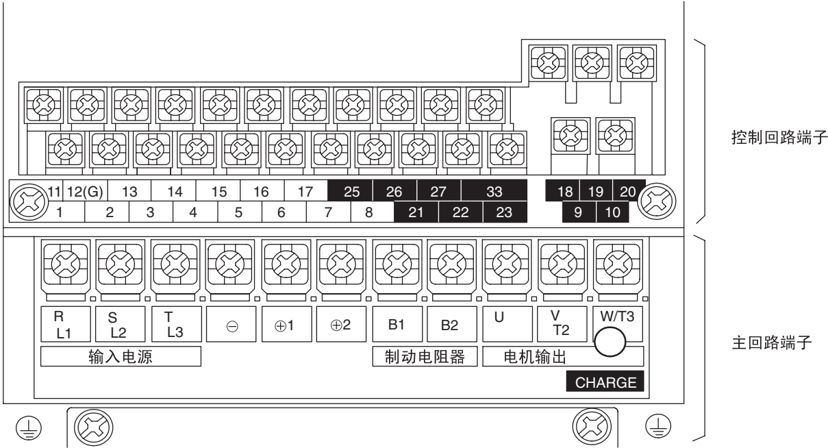
图 1.3 端子的配备
