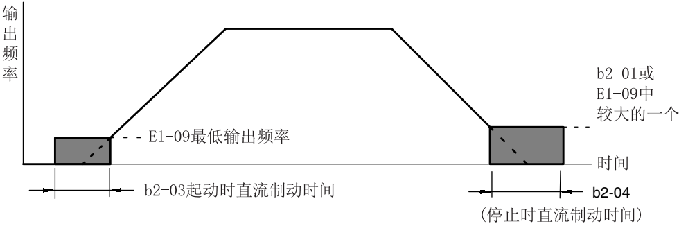
图 7.19 所示，直流制动（初期励磁）的时序图。
