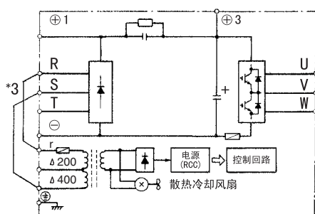
CIMR-G5A4185~4300形 (185~300kW)
