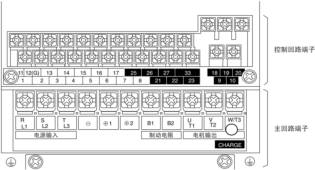
图 3.3 端子的配备
