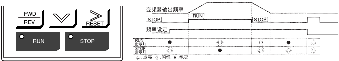
RUN STOP 指示灯, 对应有点亮, 闪烁, 熄灭表示运行状态 图 1.5 RUN STOP 指示灯的表示
