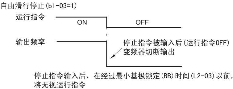
图 6.5 自由滑行停止
