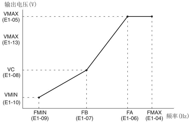
图 7.3 任意 V/f 曲线
