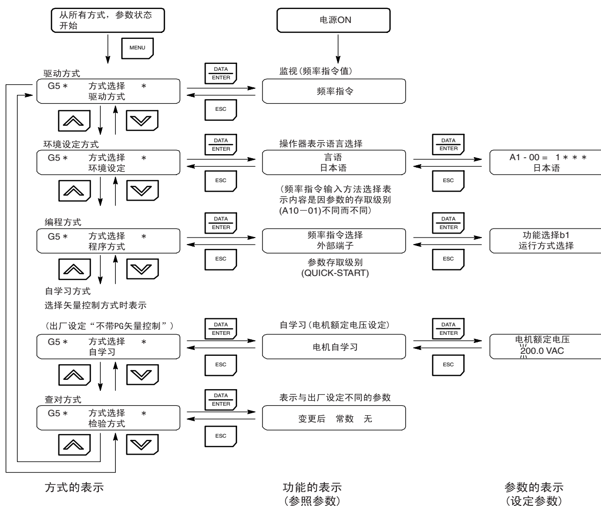
图 4.3 方式的切换
