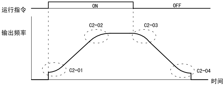
图 7.27 S 字特性功能的设定
