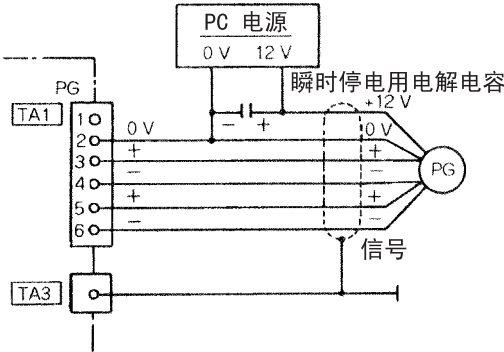
图 3. 33 PG-B2 接线例
