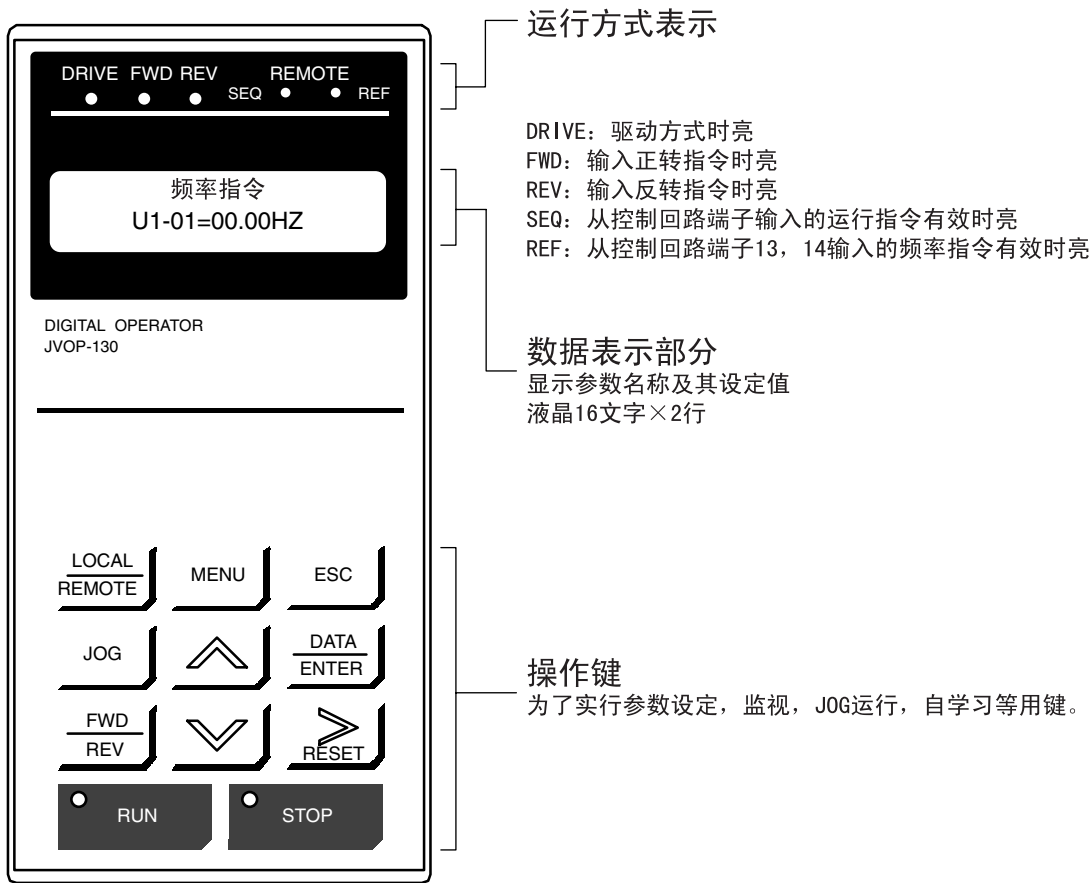
图 1.4 数字操作器（操作器）的各部名称和功能
