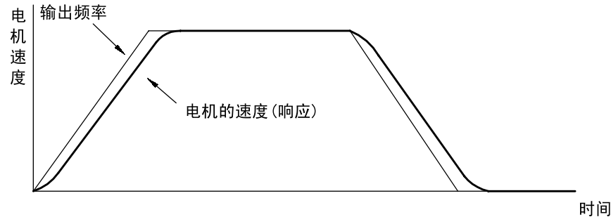
图 6.23 观测波形举例
