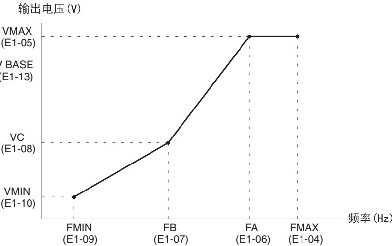
图 6.11 任意 V/f 曲线
