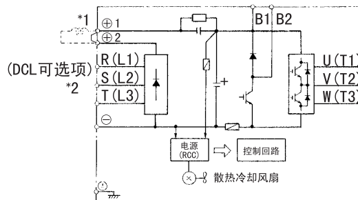
CIMR-G5A42P2~4015形 (2.2~15kW)
