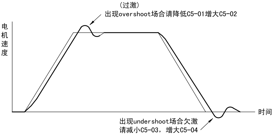
图 6.24 增益的调整
