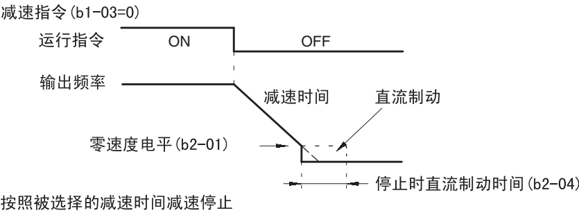
图 6.4 减速停止
