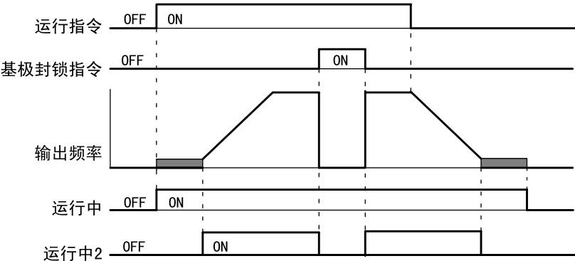
图 7.43 运行中的时序图
