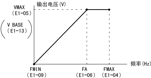
图 7.17 V/f 曲线的调整
