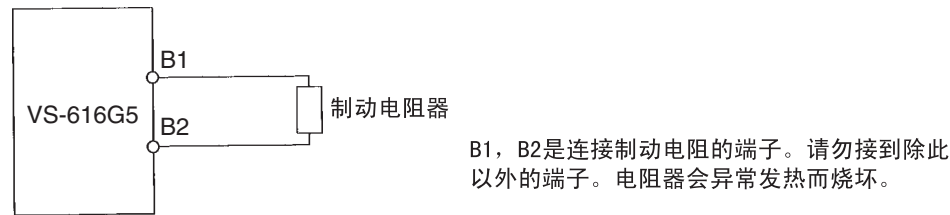
图 3.14 制动电阻器的连接
